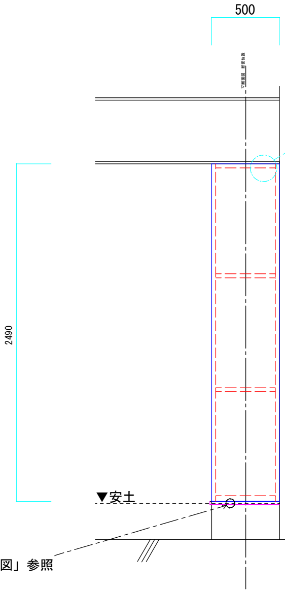
袖壁 立面図 (弓道場側からの的場側方向)
