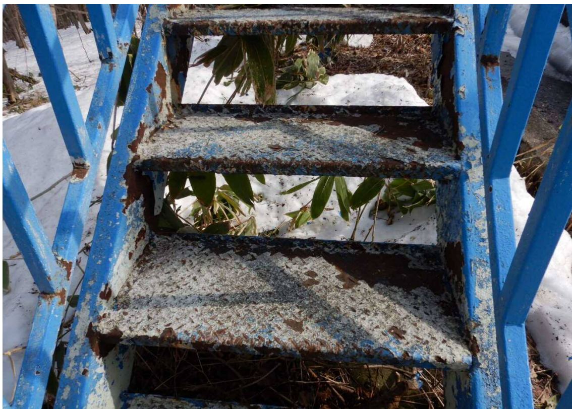
腐食・破損状況（横断橋②）
