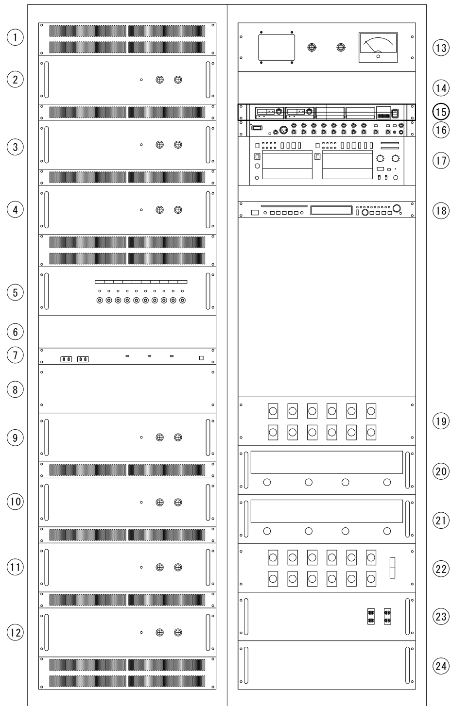
機器収納架 実装図 (参考)
