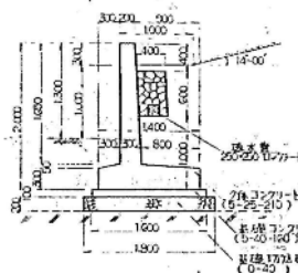
A717断面図 S=1:40
