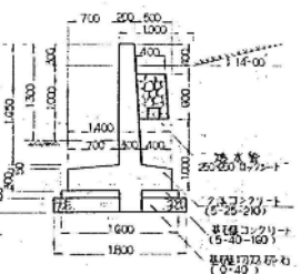
B917断面図 S=1:40
