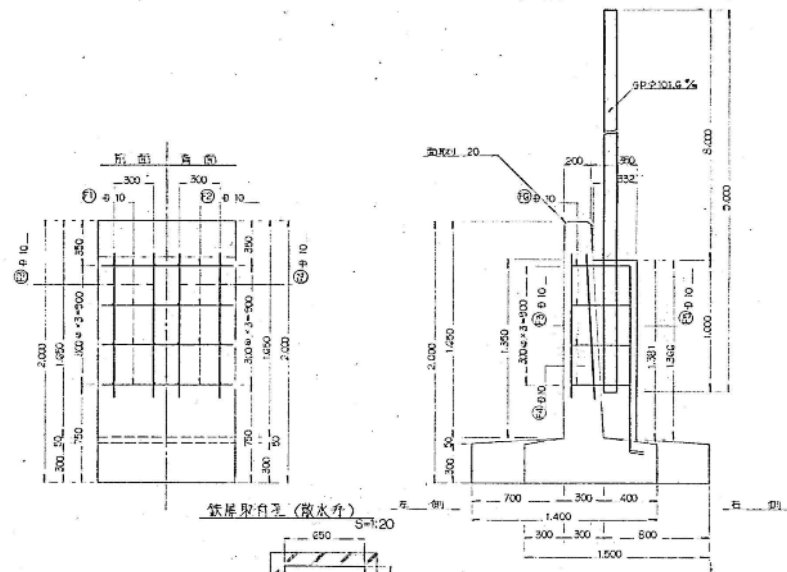
B917RC 擁壁 H=2.000 B=1.400 変形断面
