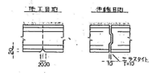
RC 擁壁 目地詳細図 S=1:10
