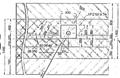
平面図 S=1:20
