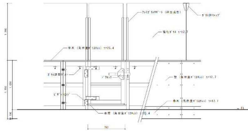
選手一般出入口 立面図 S=1:20
