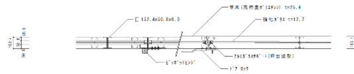
選手出入口 平面詳細図 S=1:20
