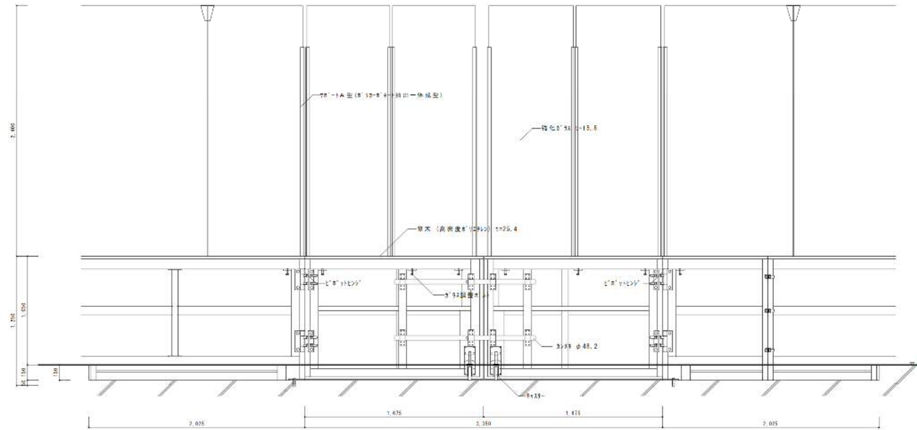
マシン出入口 立面図 S=1:20
