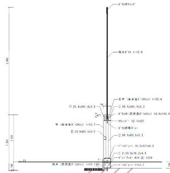
7A271 断面図 S=1:20
