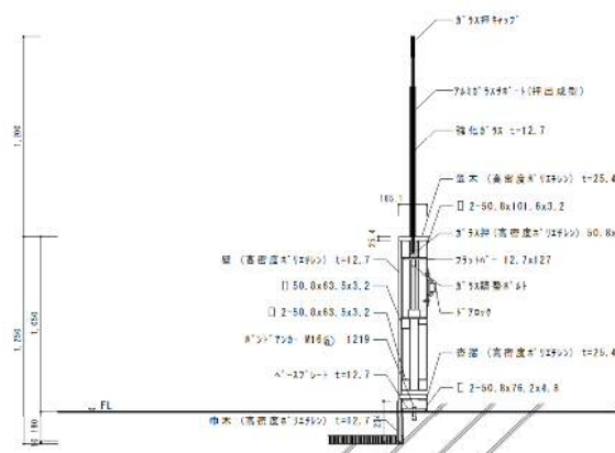
7A272出入口 断面図 S=1:20
