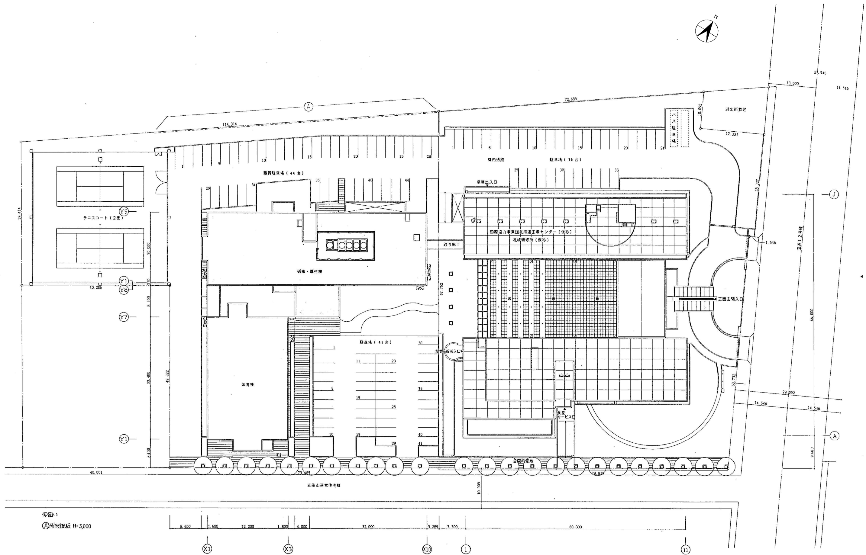
リフレサッポロ 配置図
