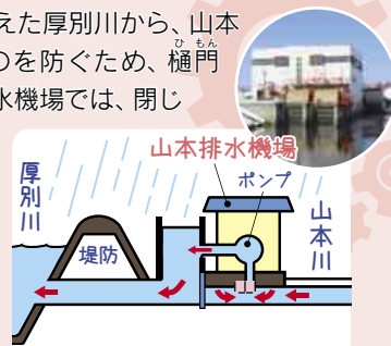
※簡略図
