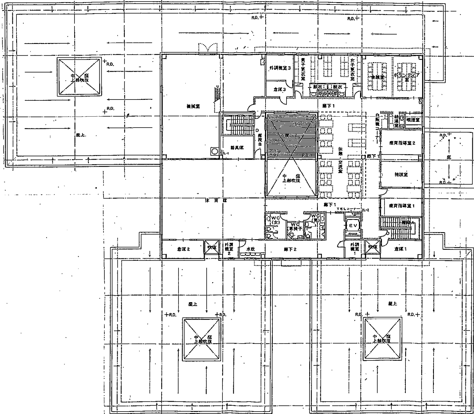
札幌市自閉症者自立支援センター及び札幌市自閉症・発達障害支援センター2階図面
