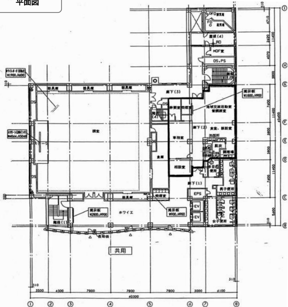
夜間急病センター・保健所他複合施設 5階平面図
