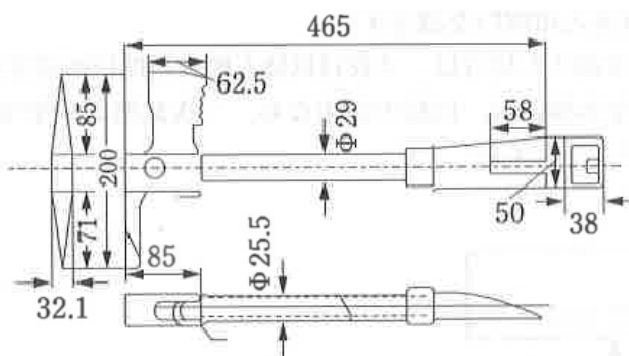
図4 破壊器具
