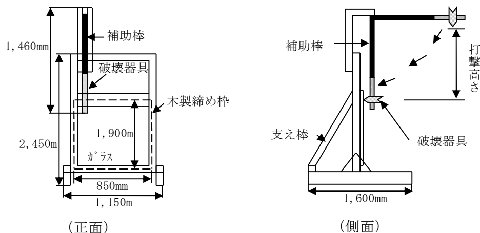
図1 本体
