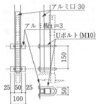
図5 固定方法
