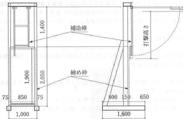
図1 本体
