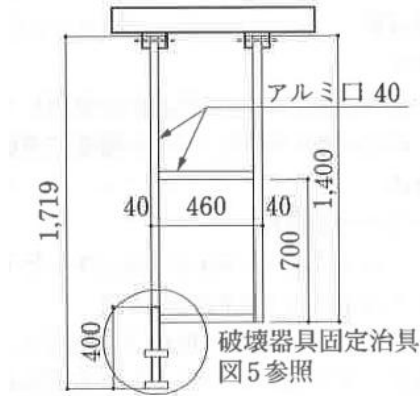
図3 補助棒
