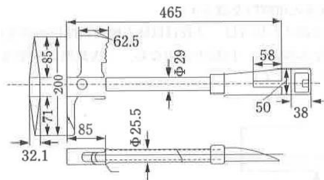
図4 破壊器具
