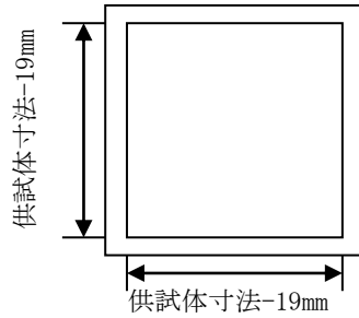
図2 締め枠
