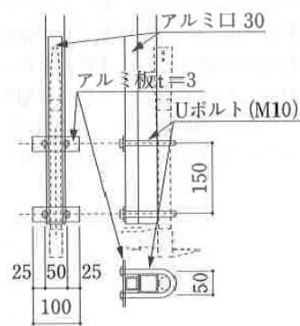
図5 固定方法
