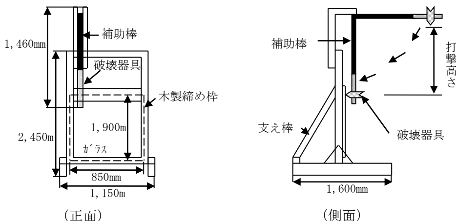
図1 本体
