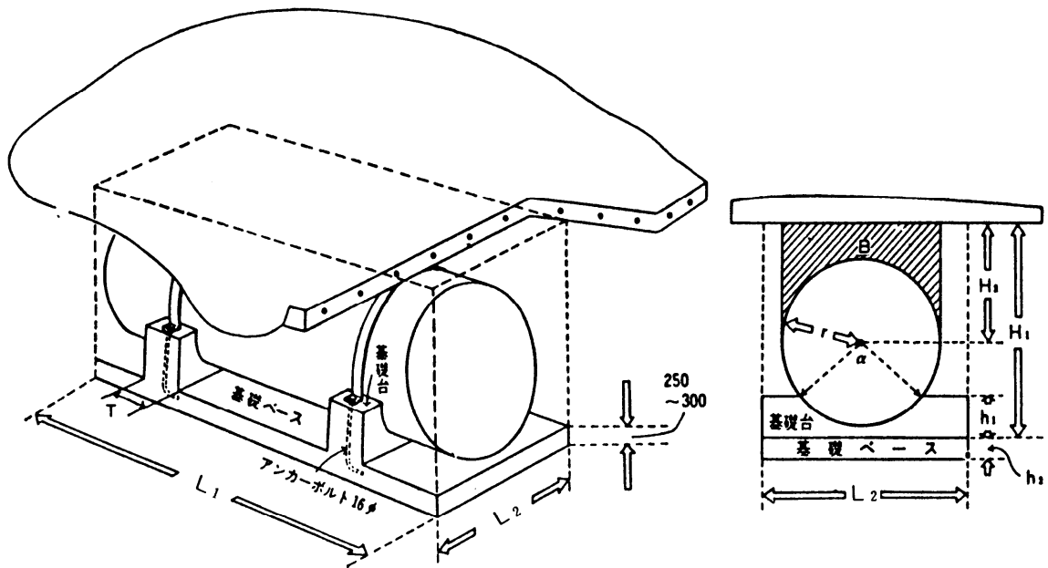
第9-10図 固定方法の例図
