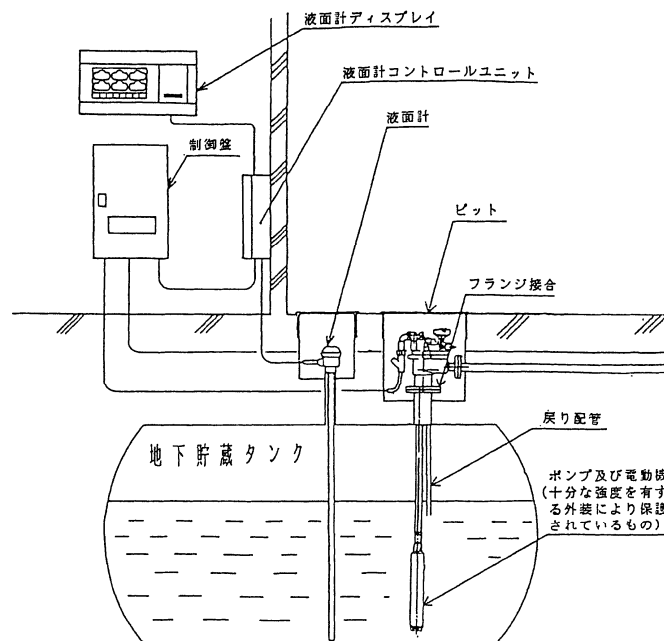
第9-2図 油中ポンプ設備の設置例
