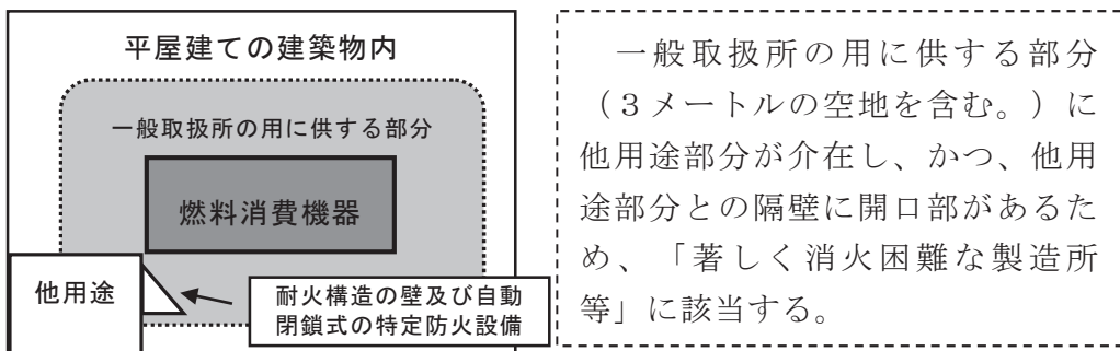
第20-2-2図 設備単位の一般取扱所で他用途部分が介在する場合
