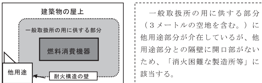
第20-3-2図 屋上の設備単位の一般取扱所で他用途部分が介在する場合
