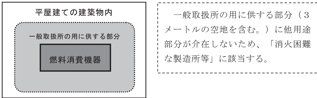
第20-2-1図 設備単位の一般取扱所で他用途部分が介在しない場合
