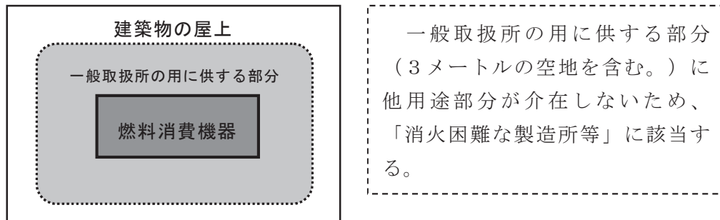
第20-3-1図 屋上の設備単位の一般取扱所で他用途部分が介在しない場合
