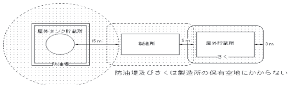
第5－2図 保有空地の例
