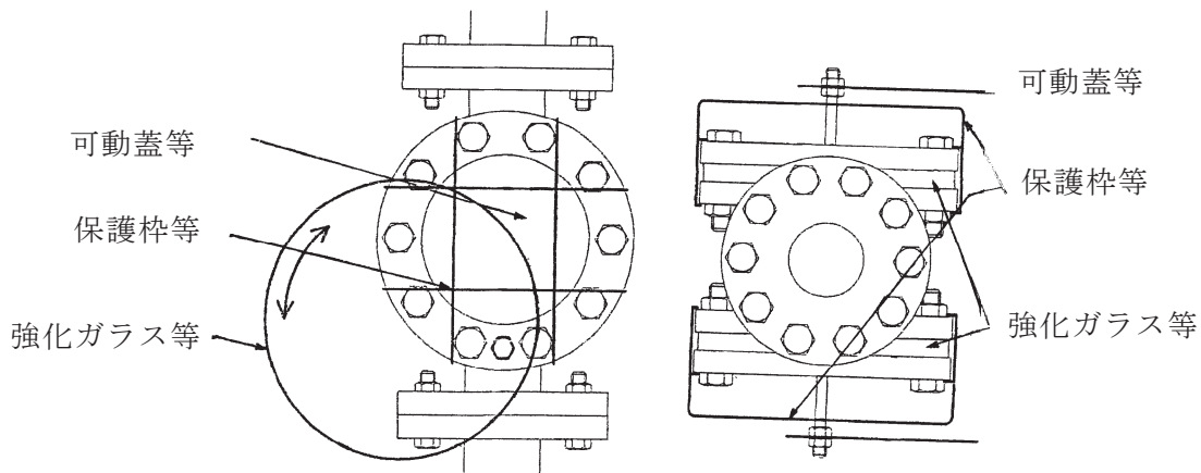
第5-18図 容易に破損しない構造例
