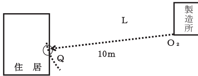
第5-1図 防火上有効な塀
