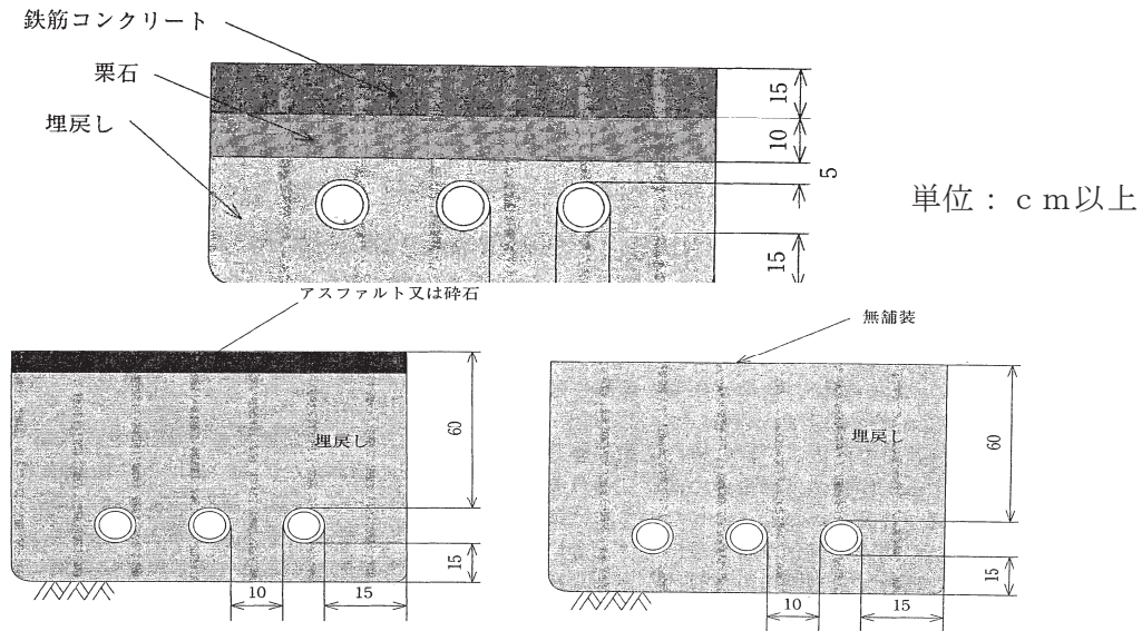
第5-17図 埋設構造例
