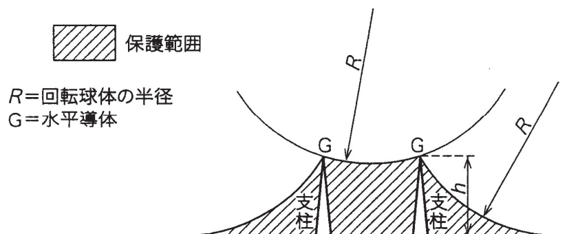
第5-7図 受雷部システムの例（回転球体法による例）
