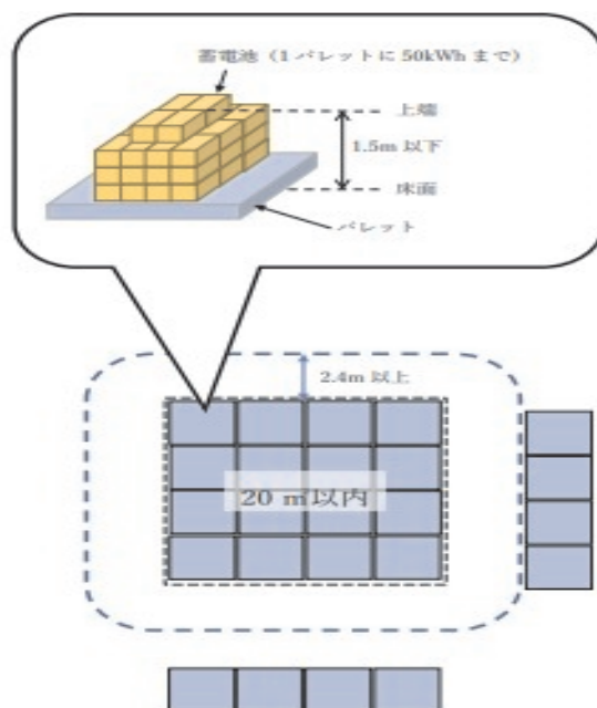
危険物の規制に関する規則第16条の2の8第2項第5号ハの貯蔵方法（例）
