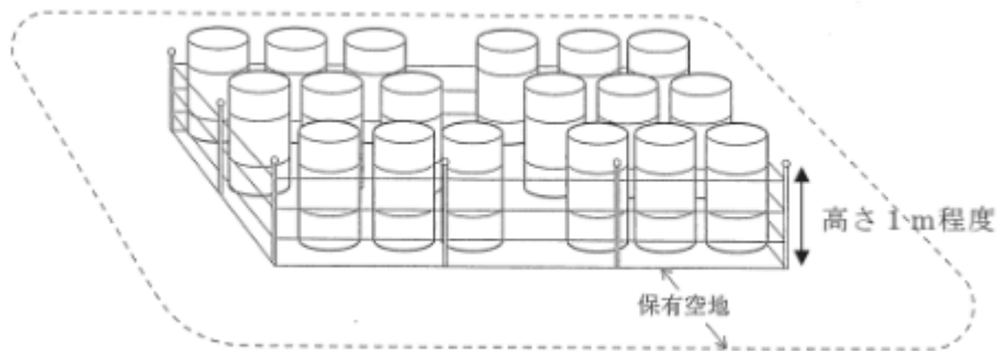
第12-1図 さくを設けた場合の例
