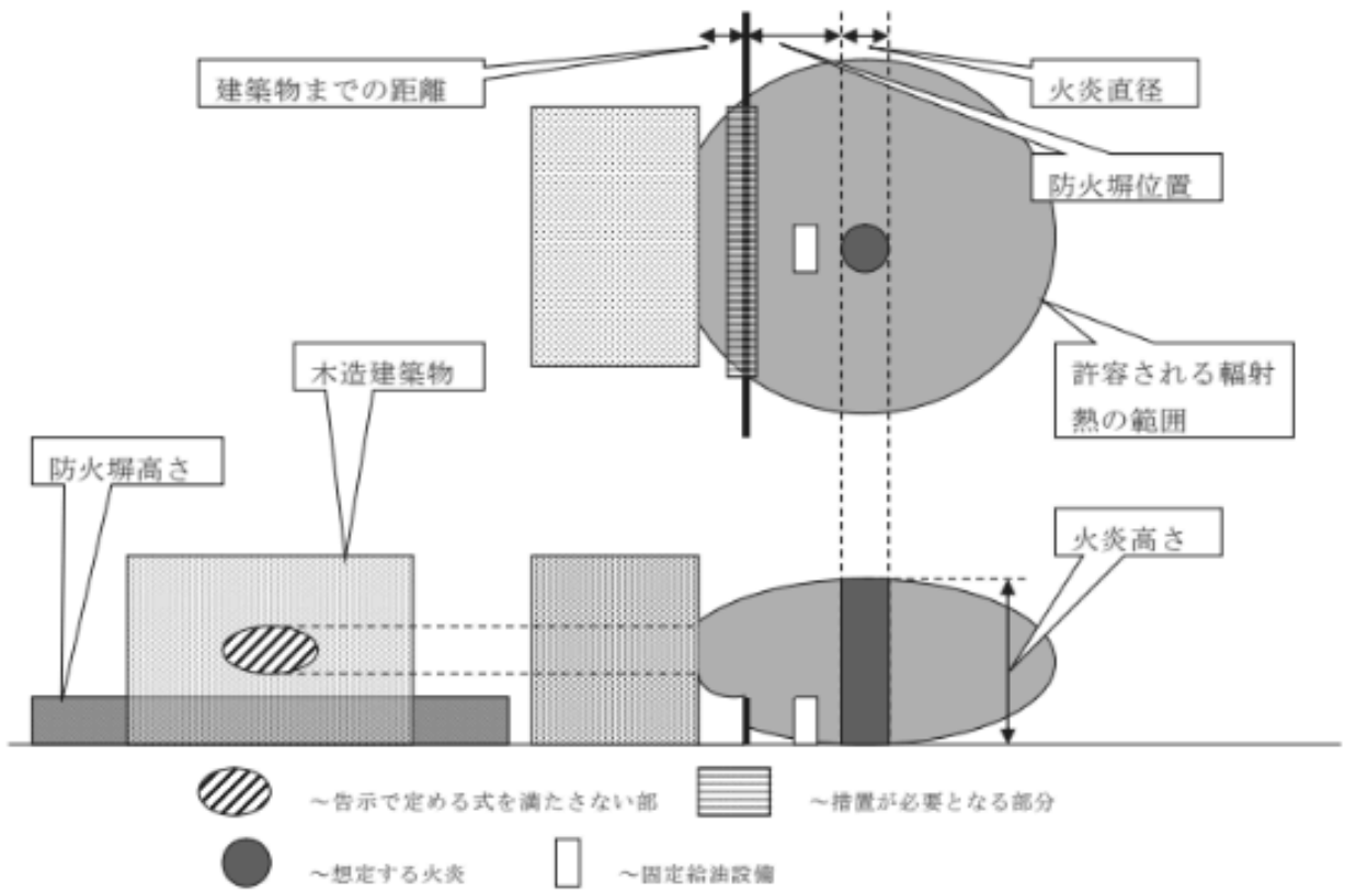
第1-5-1図 火災想定イメージ
