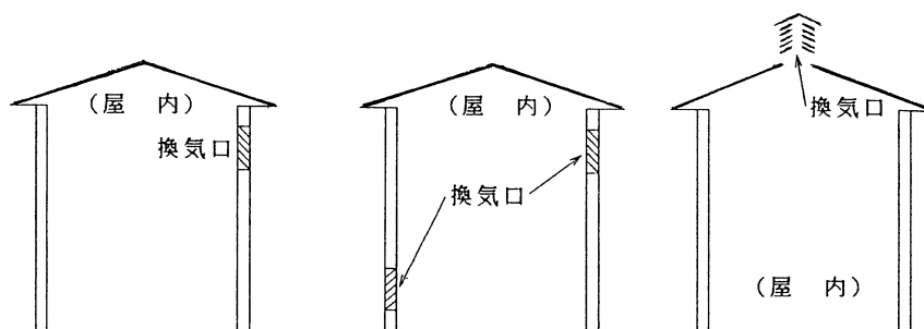
第 17-1 図 自然換気設備の例
