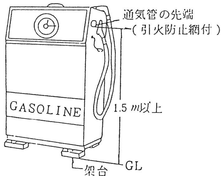
第10-1図 通気管の高さ
