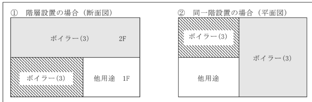
第15-2-1図 同じ取扱形態のものを2施設として設置した例
