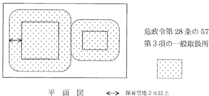
第15-6-7図 危政令第19条第2項の1施設とした例 (設備単位の規制)
