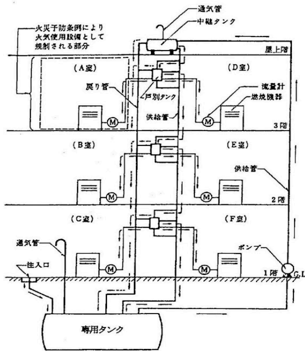
第15-30図 中継タンクを有する方式の燃料系統図 (系統例1)
