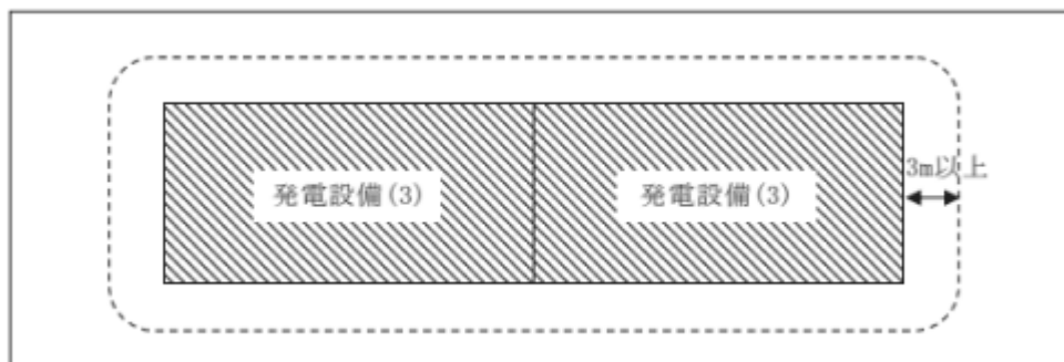
第15-4-1 図 同じ取扱形態をまとめて1施設として設置した例 (それぞれの発電設備の指定数量の倍数を合算した値は10未満)
