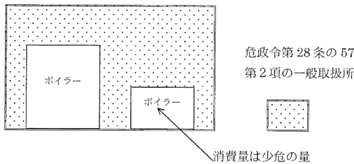
第15-6-6図 危政令第19条第2項の1施設とした例 (区画室単位の規制)
