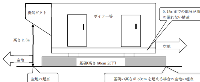
第6-6図 空地の起点の取り方
