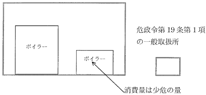
第15-6-5図 危政令第19条第1項の1施設とした例
