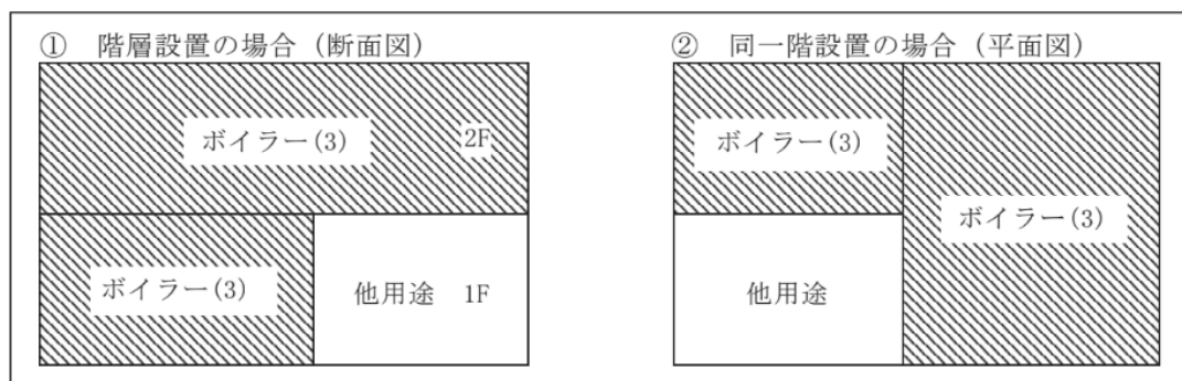
第15-2-2図 同じ取扱形態のものを1施設として設置した例
