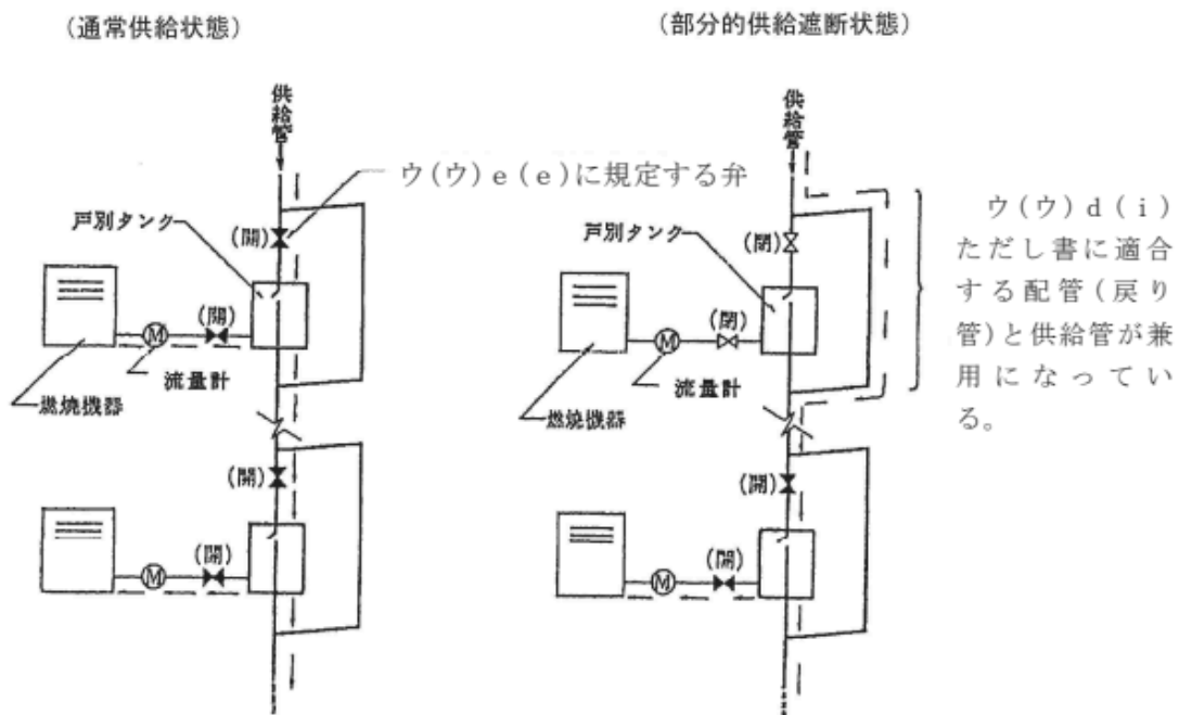
第15-34図 燃料供給系統詳細図 (系統例2)
