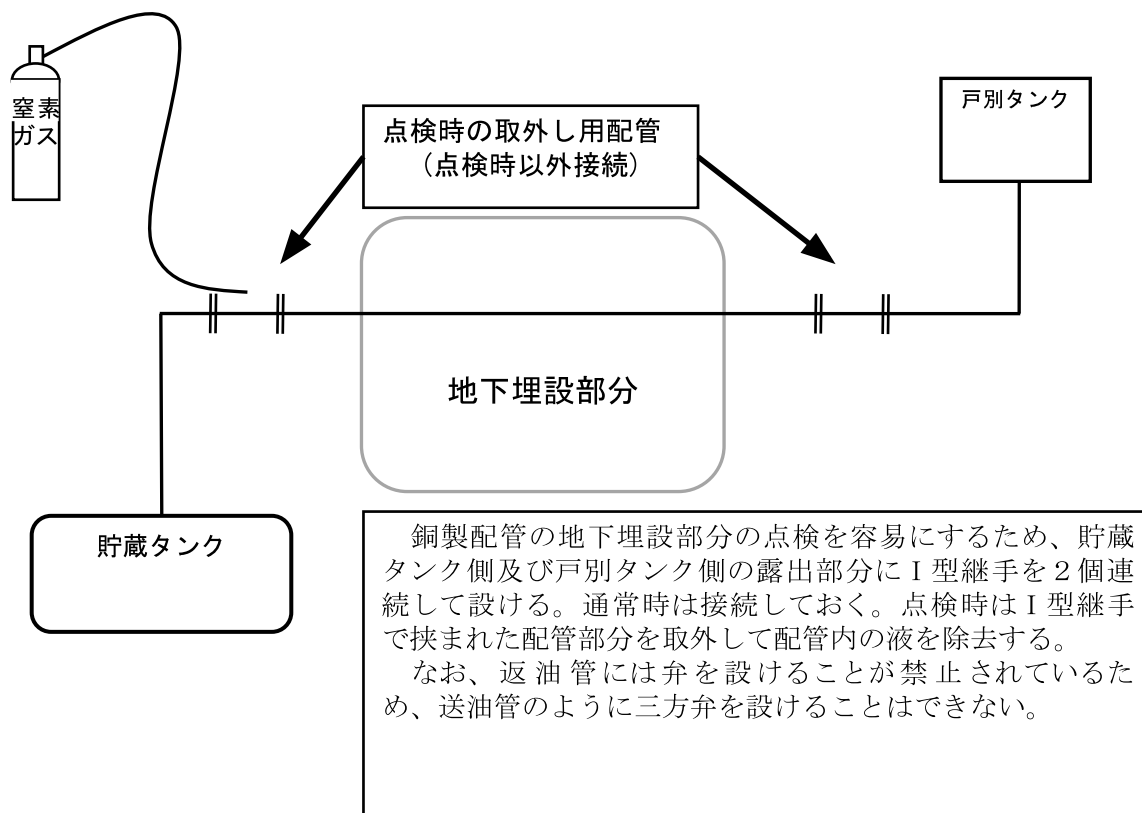
図2 (返油管の場合)
