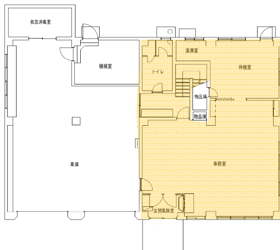
1 階 平面図
