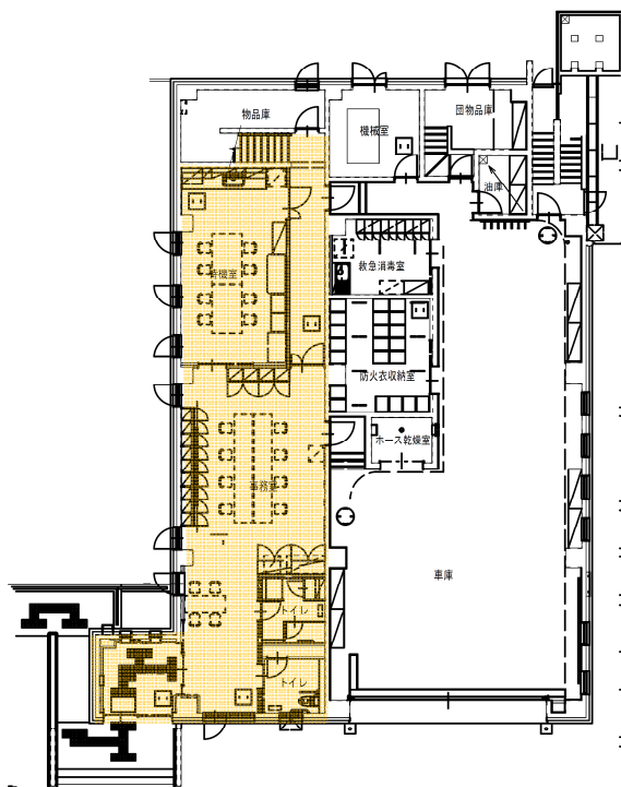
1 階 平面図
