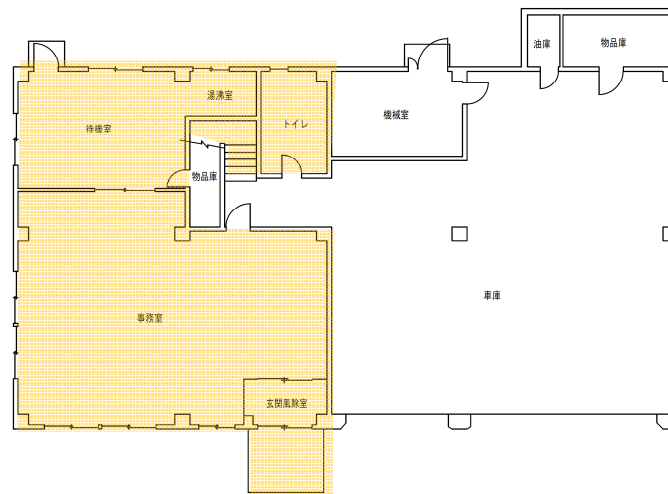
1 階 平面図
