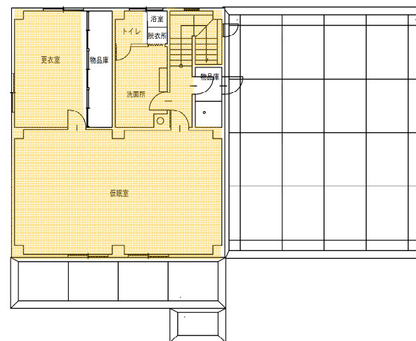
2 階 平面図
