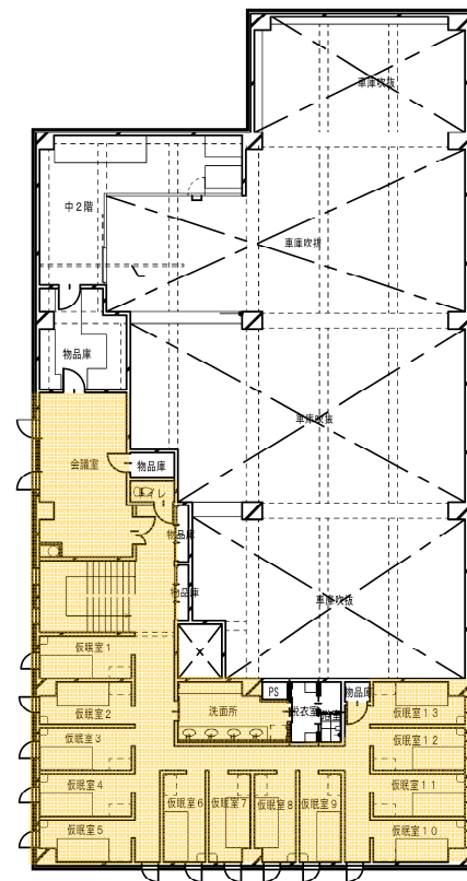
2 階 平面図
