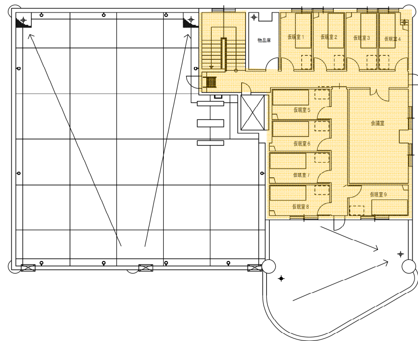
2 階 平面図
