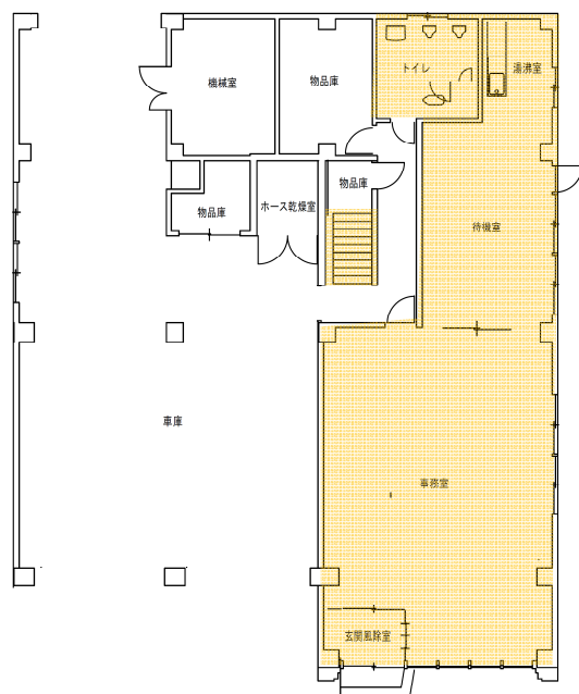
1 階 平面図
