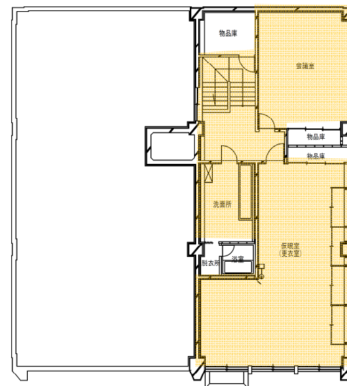
2 階 平面図
