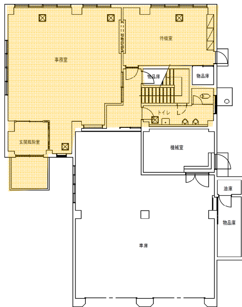
1 階 平面図
