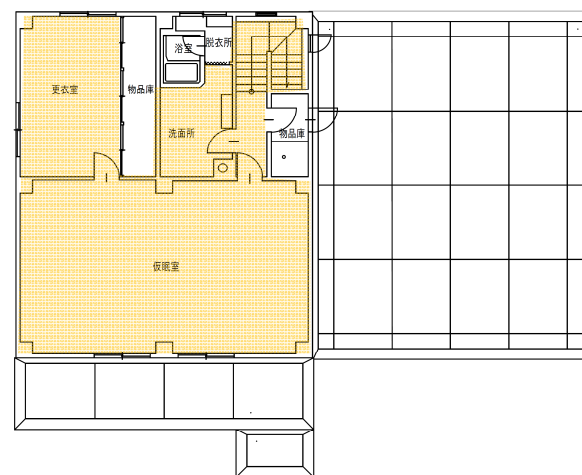
2 階 平面図
