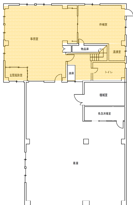
1 階 平面図
