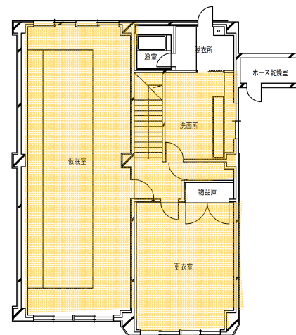
2 階 平面図
