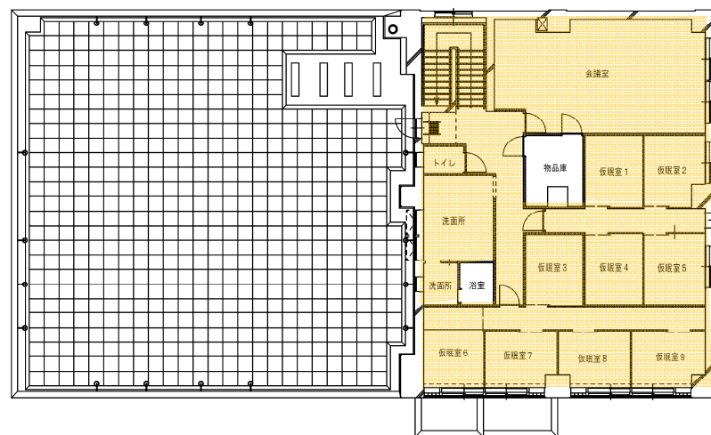
2 階 平面図
