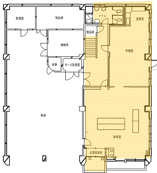
1 階 平面図
