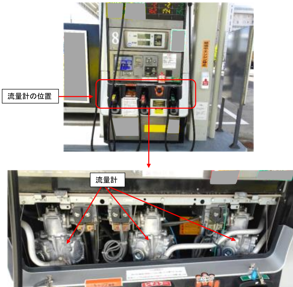
【流量計の例①】
