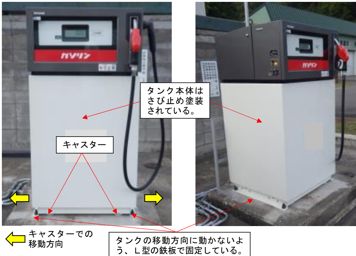
【簡易タンクの固定例①】
