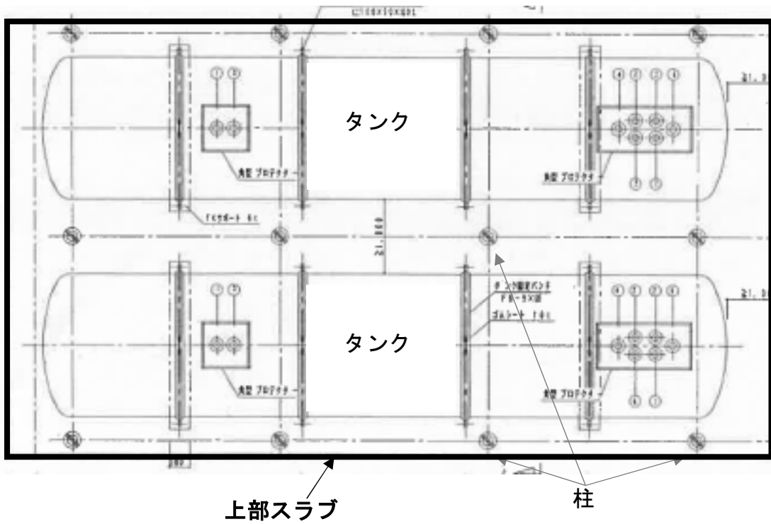
【給油取扱所の平面図の例】
