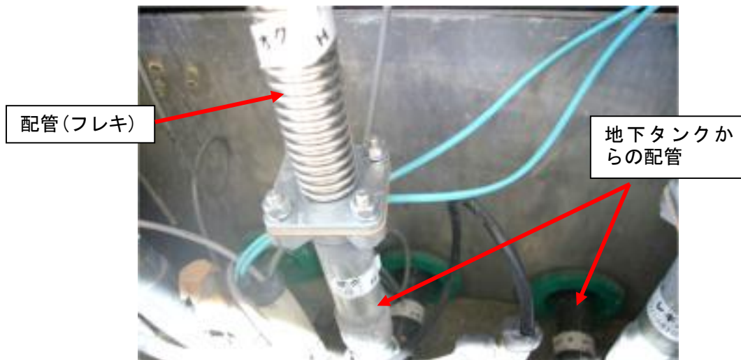
【ピット内】
