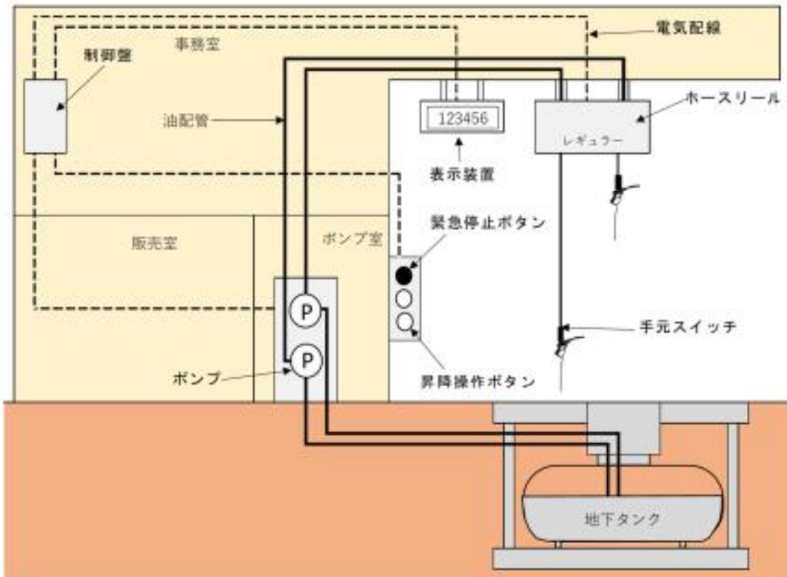
【懸垂式固定給油設備の系統図例】
