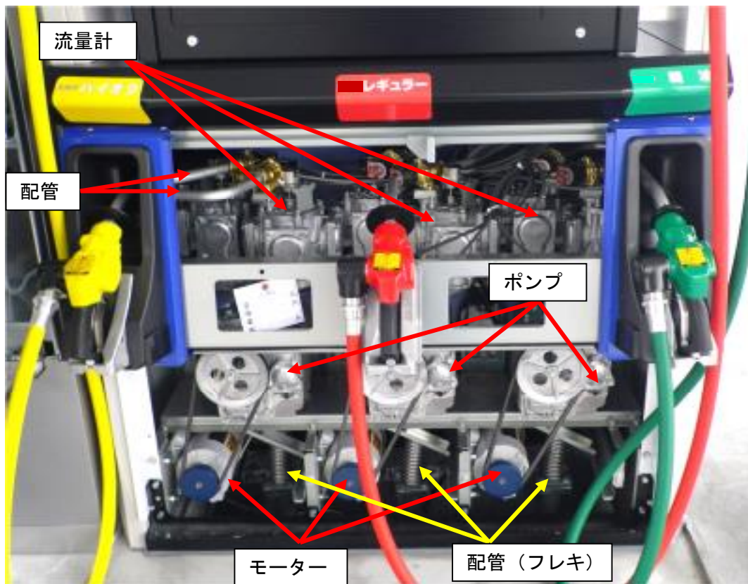
【上の計量機のパネルを外した状態】
