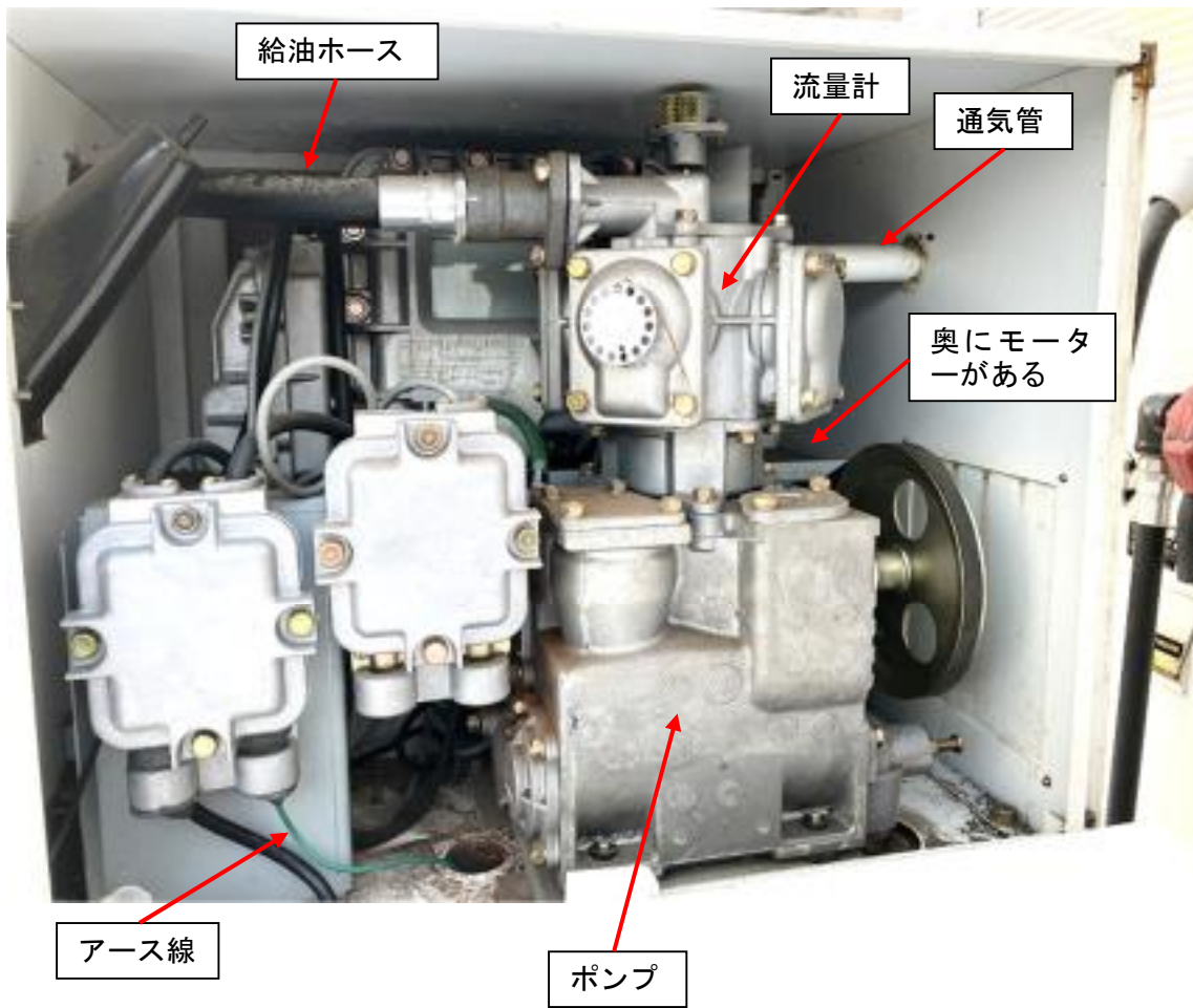
【簡易タンクの例（簡易タンク上部の給油設備）】
