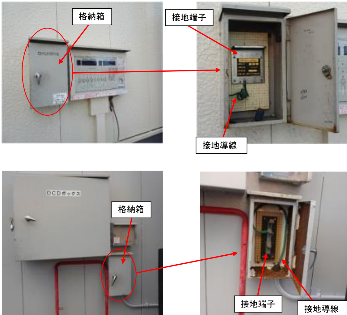
【接地電極の例】
