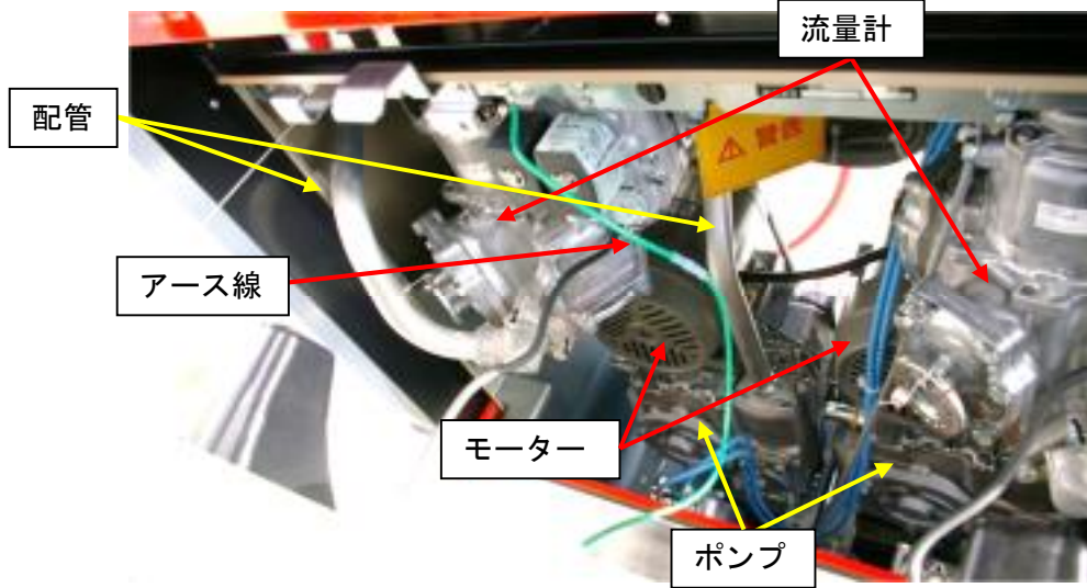
【計量機下部】
