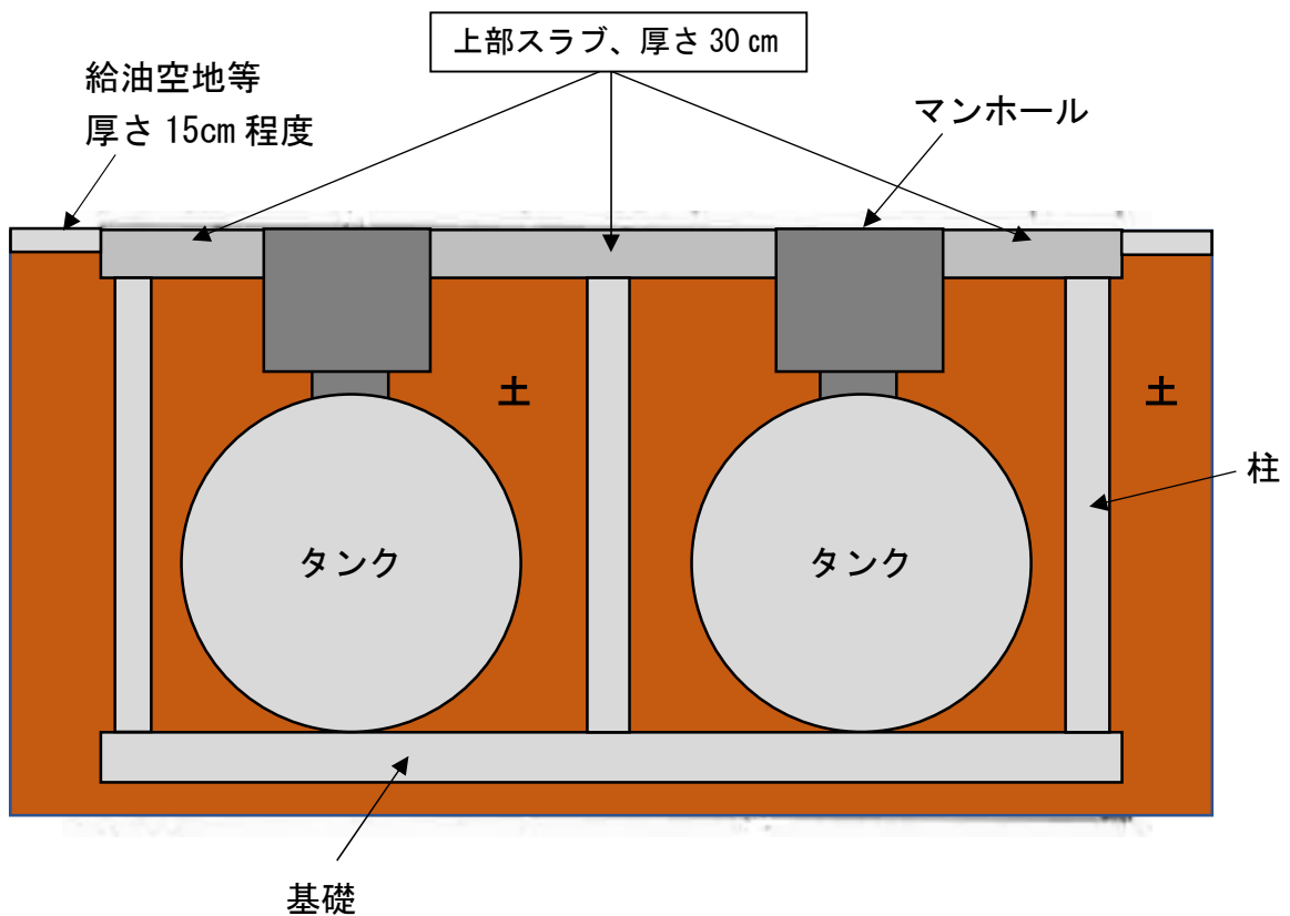
【タンク埋設のイメージ図（断面）】
