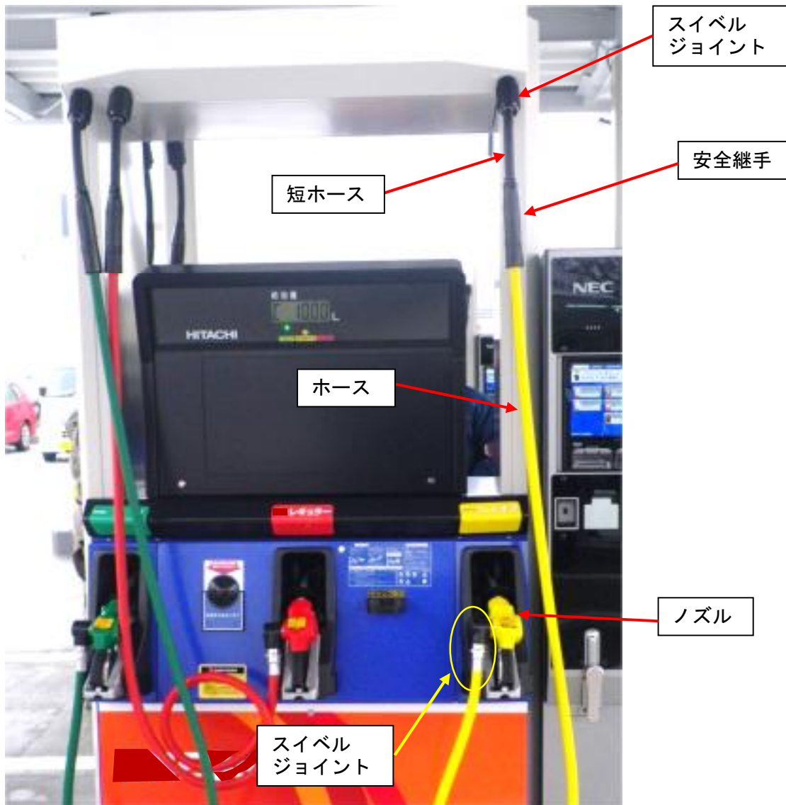
【各部の名称、例①】
