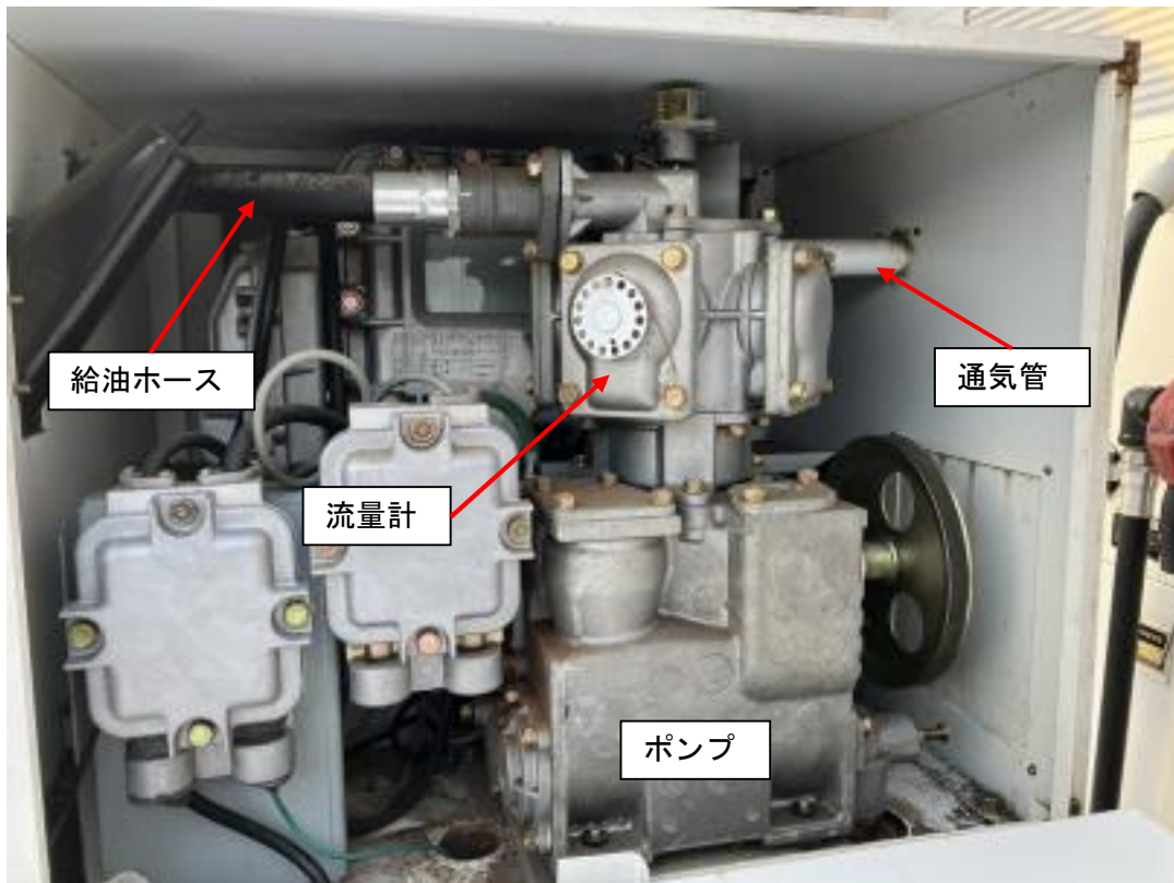
簡易タンクの上部カバーを取り外したところ
