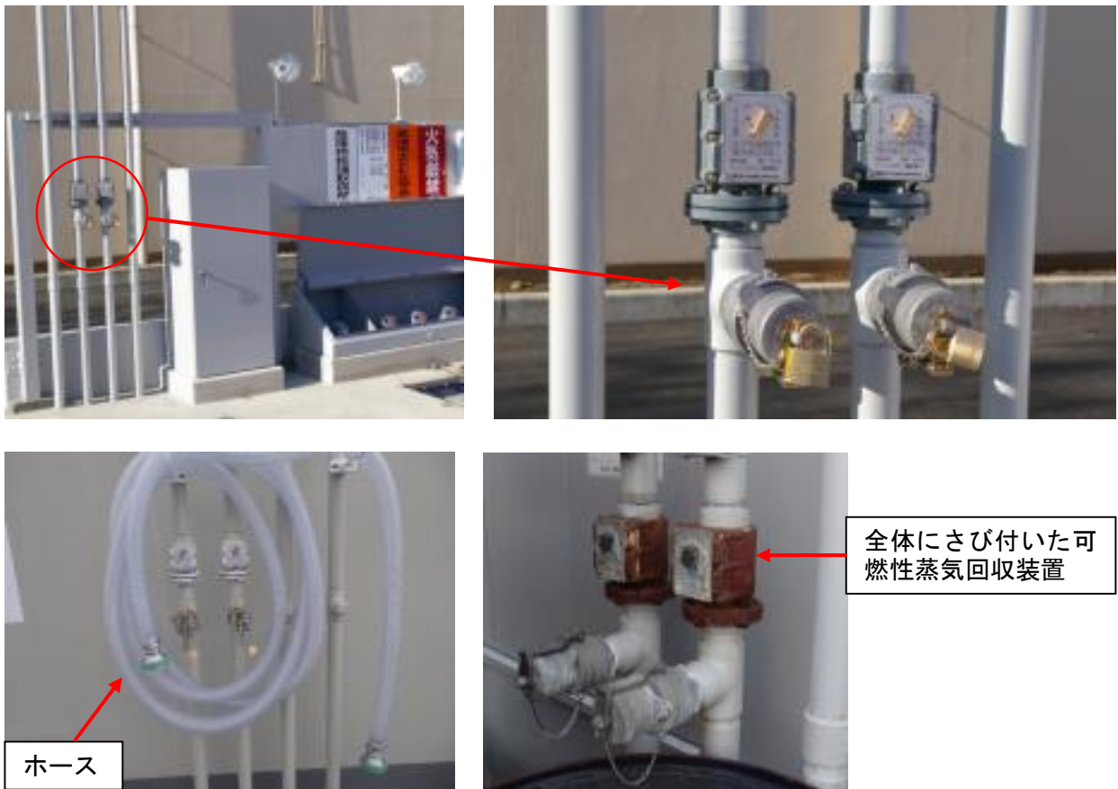
【可燃性蒸気回収装置の例】
