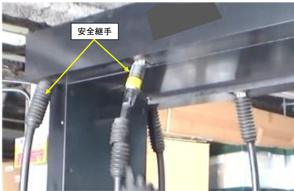
【ホース接続部の安全継手の例】
