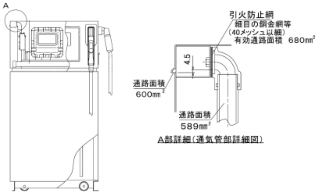
【上記簡易タンクの通気管構造図】
