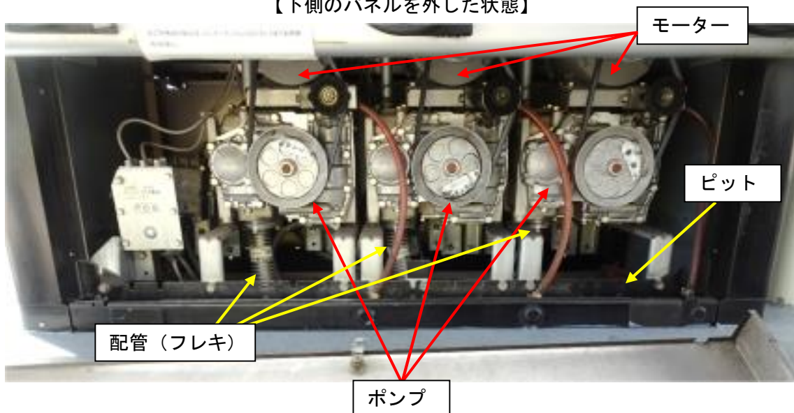
【下側のパネルを外した状態】
