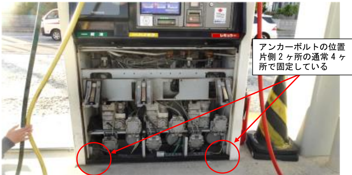
【固定ボルトの例①パネルを外した状態】
