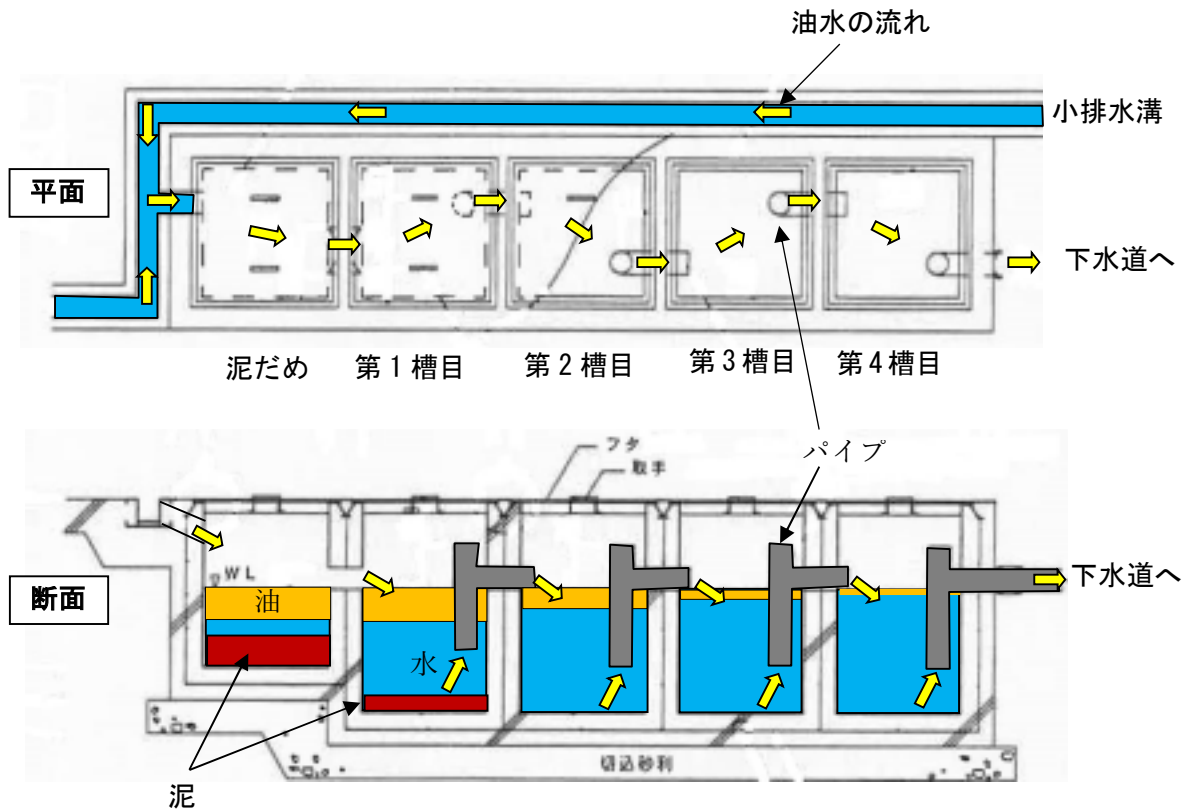
【油分離装置の例】
