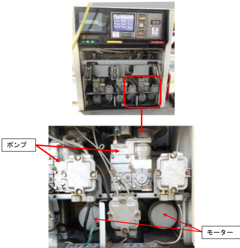
【ポンプの例①】
