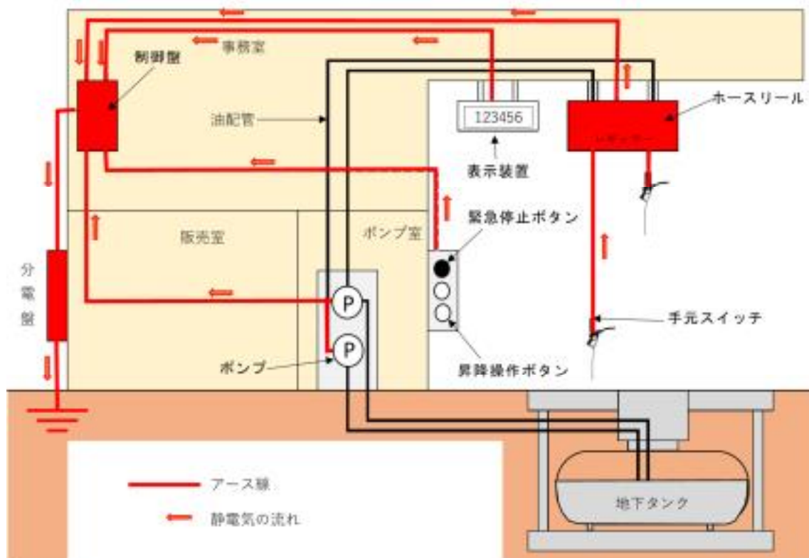
【静電気の流れ（例）】
