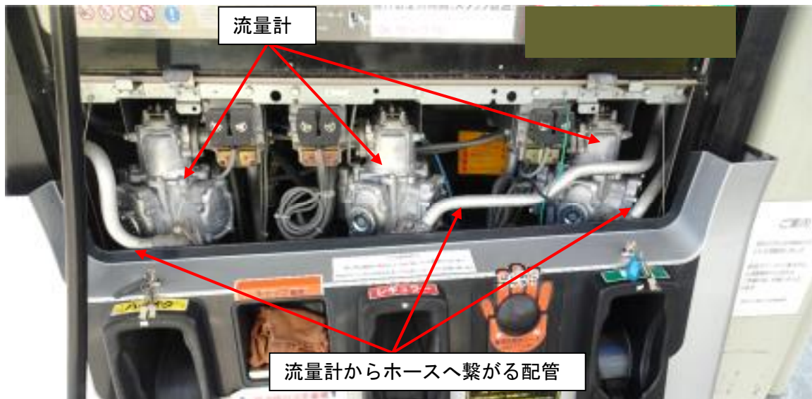
【上側のパネルを外した状態】
