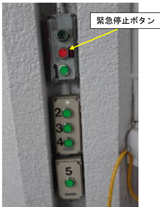
【緊急停止ボタンの例①】
