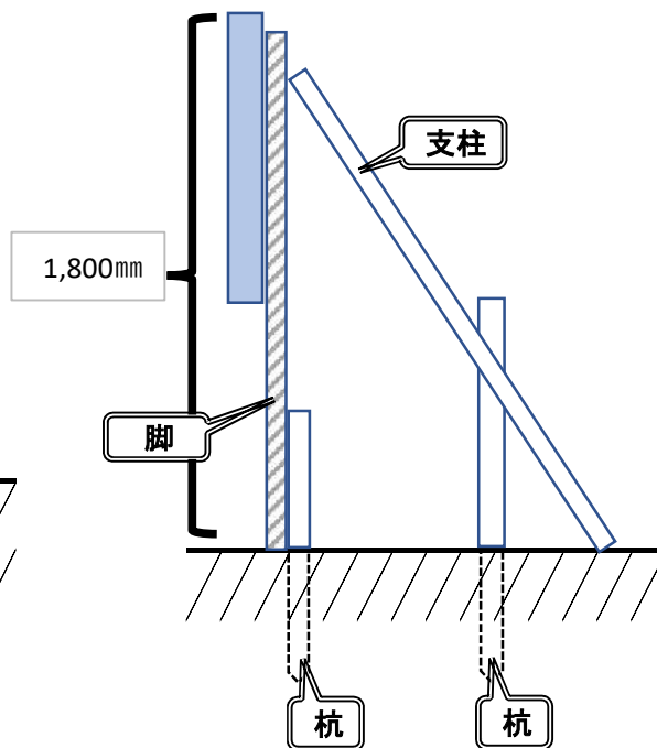
&lt; 側面図 &gt;
