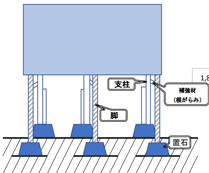
&lt;正面図&gt;
