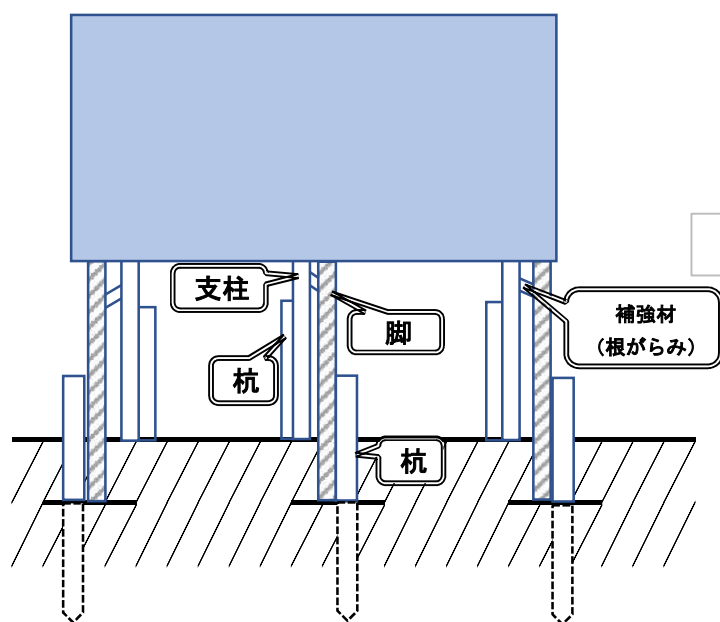
&lt; 正面図 &gt;
