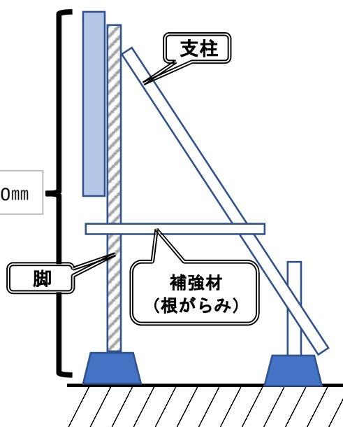
&lt;側面図&gt;
