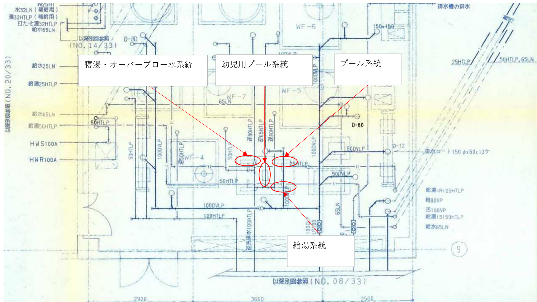
プレート式熱交換機パッキン交換位置図P-2-1
