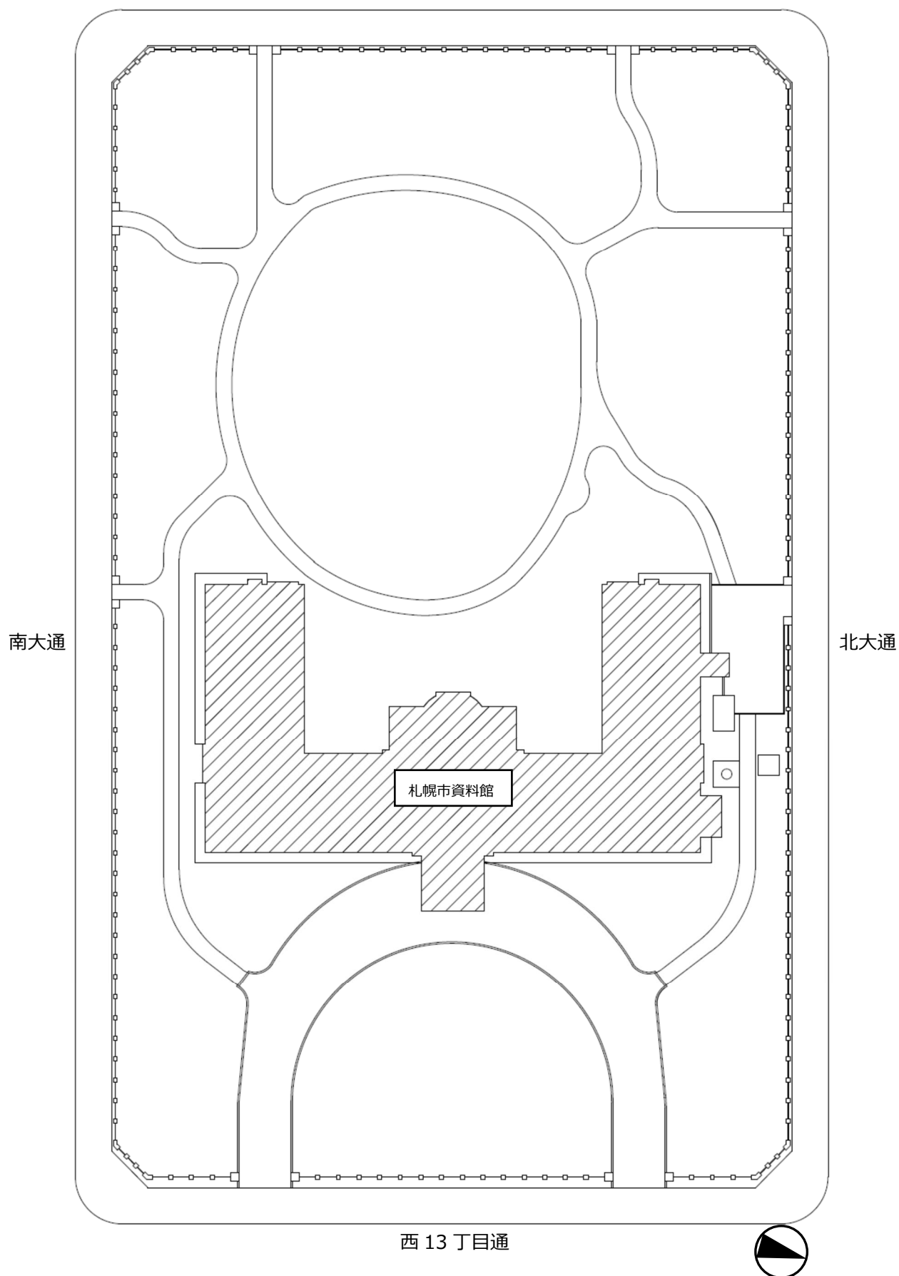
配置図 S=1:500
