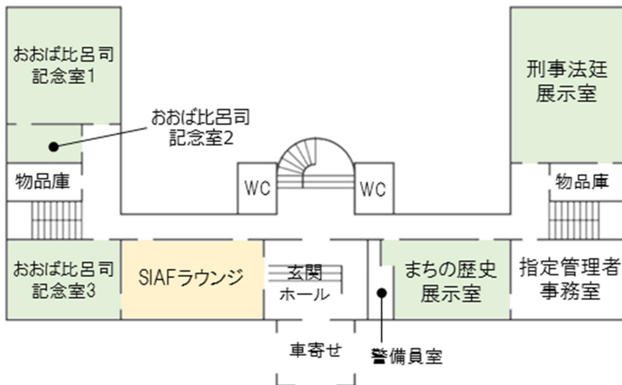
1 階平面図 S=1:300
