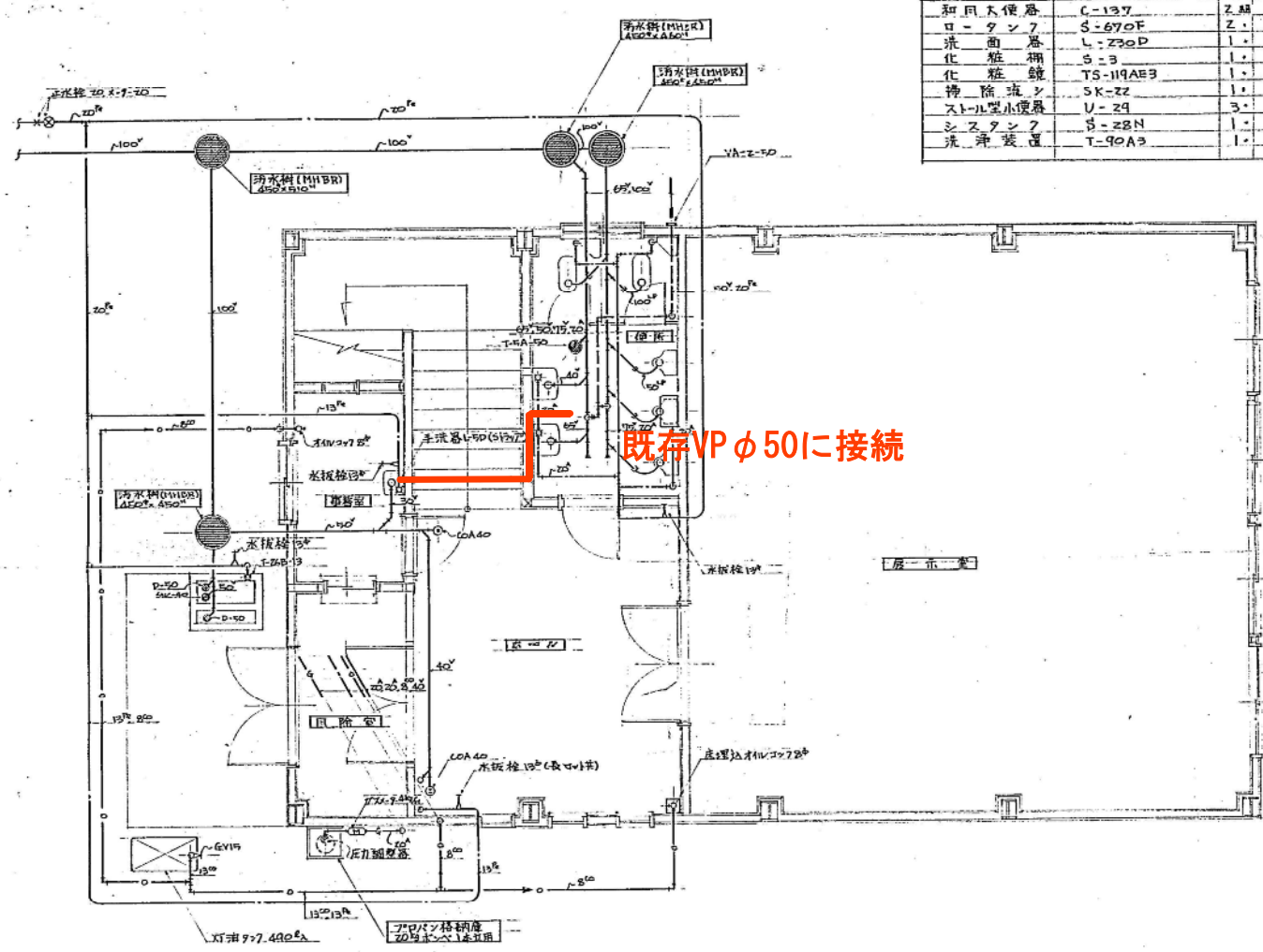
I階平面図 S 1:50
