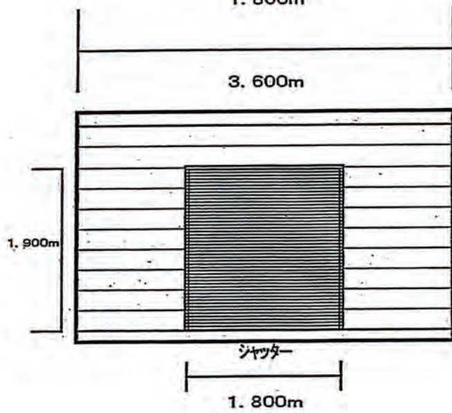
立面図 (正面)
