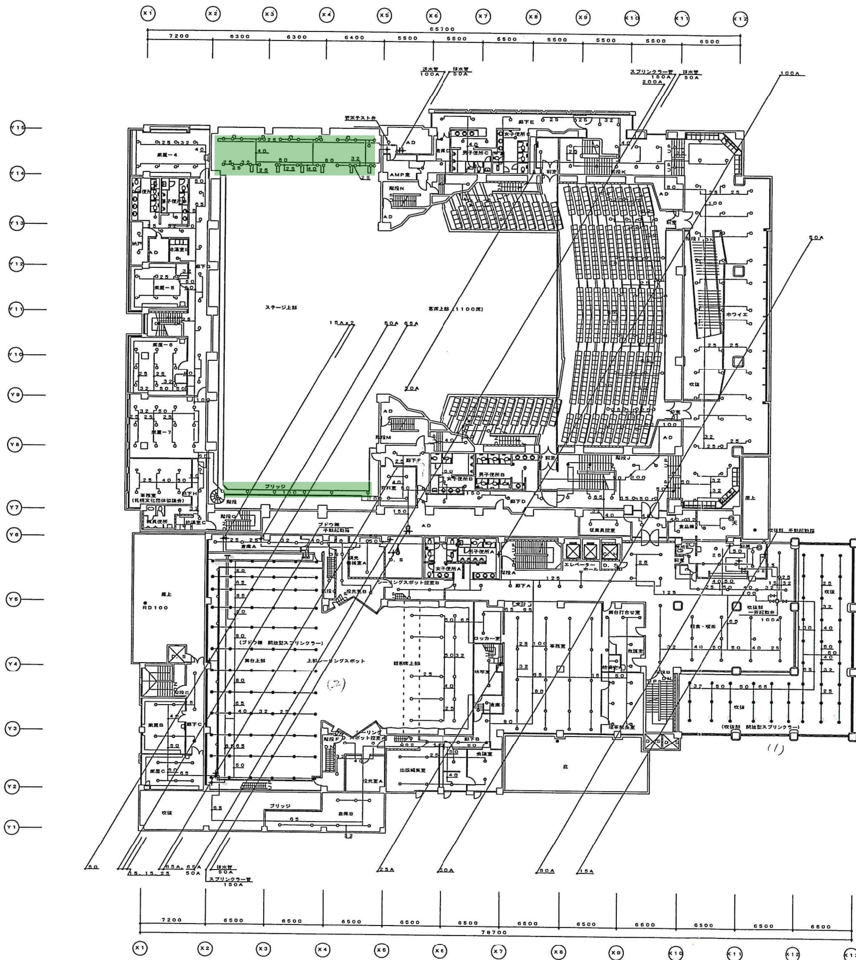
2階平面図 S=1/200
