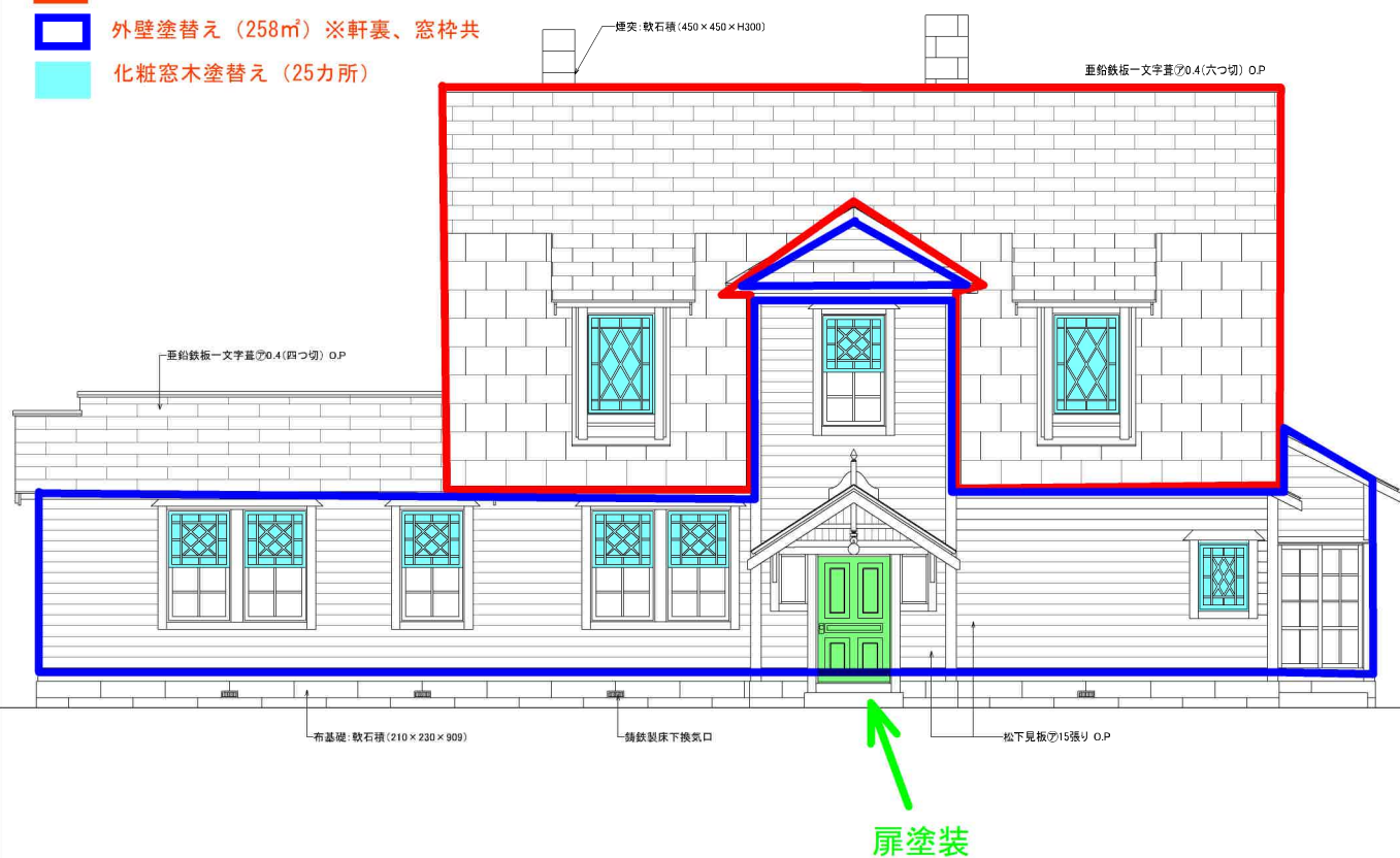
西側立面
