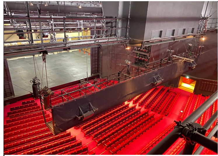
④照明トラス後方（上手側より）
