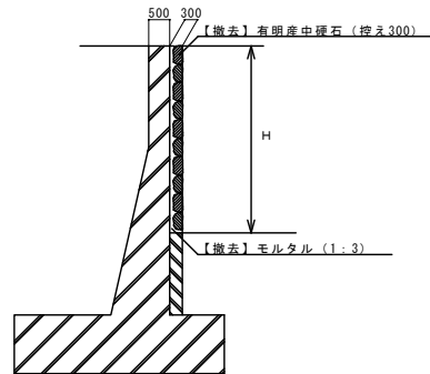
断面図 (S=1:100)
