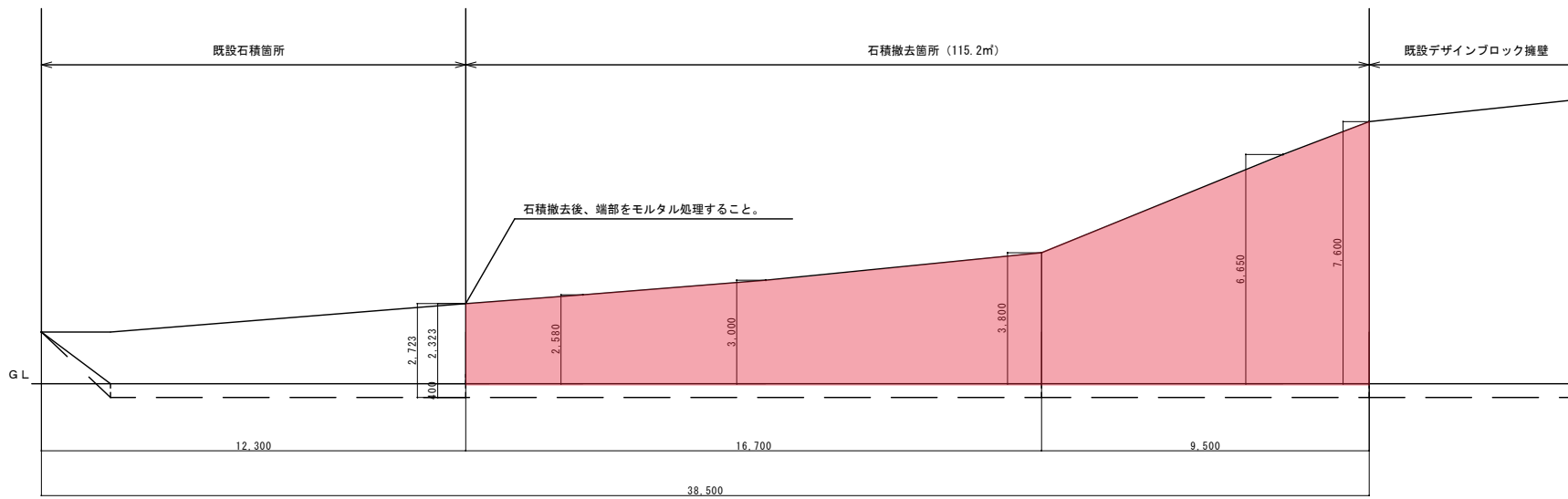
展開図 (S=1:100)
