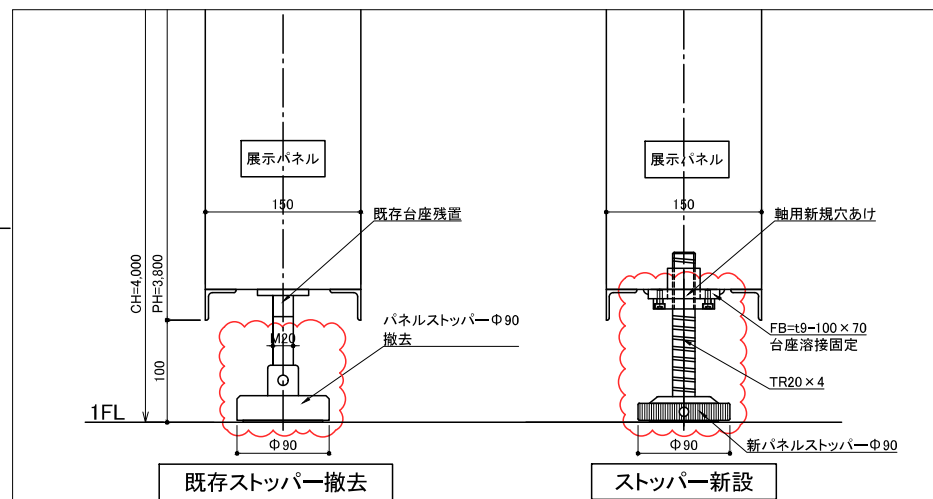
B-B断面図 A3:1/5
