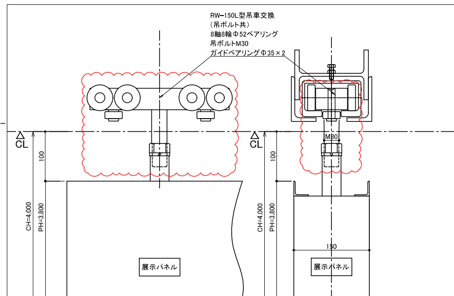
ア部拡大図 A3:1/5
