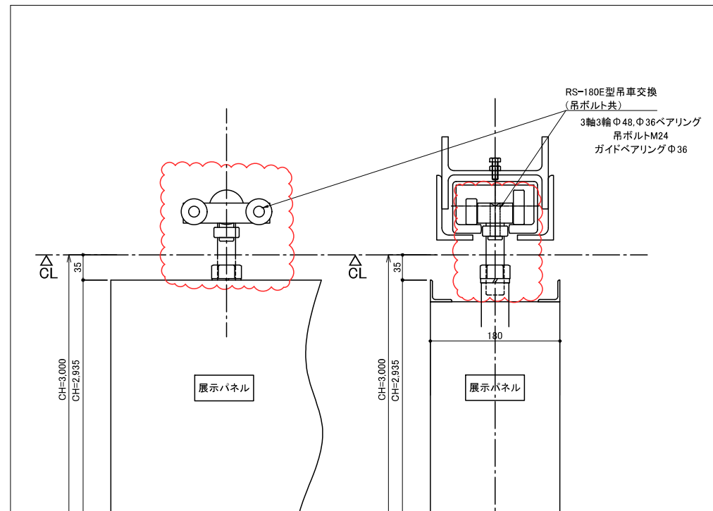
ア部拡大図 A3:1/5
