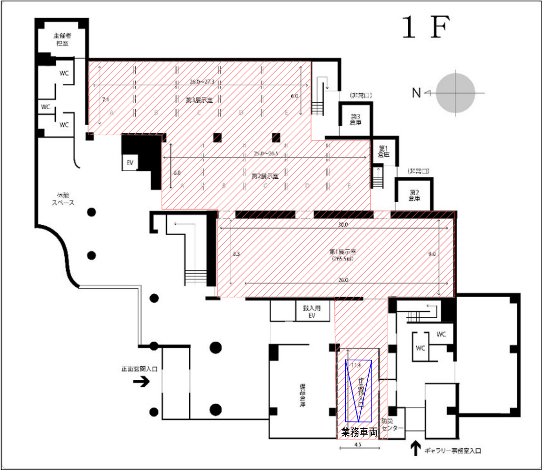
1F階平面図
