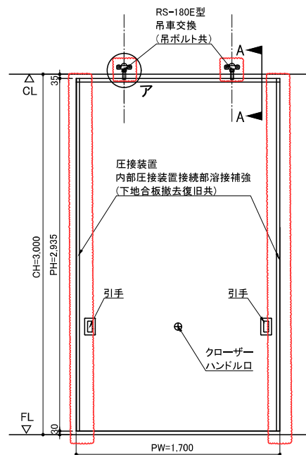
RS-180E型展示パネル 立面図 A3:1/30
