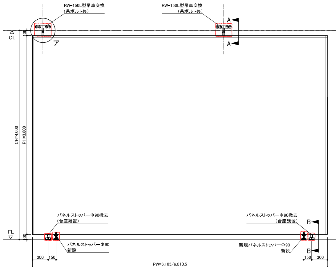
RW-150L型展示パネル 立面図 A3:1/30
