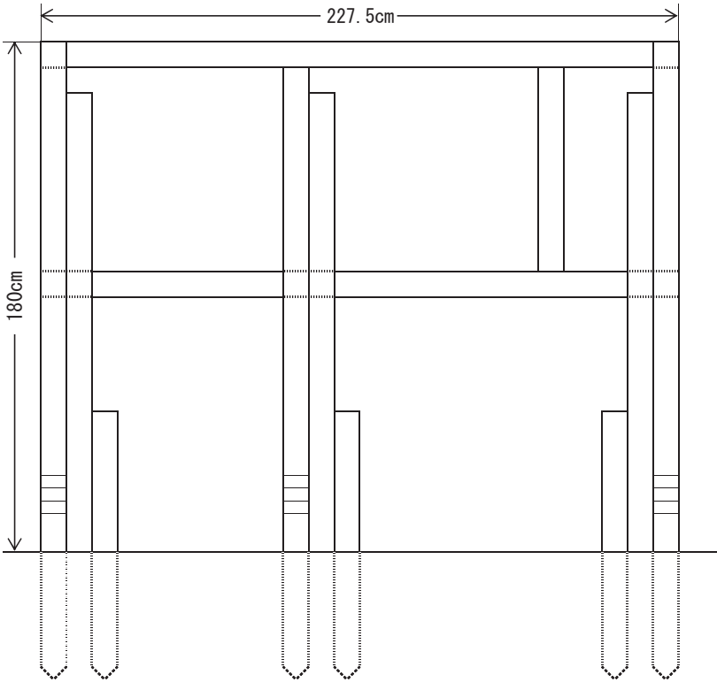
（背面図）
