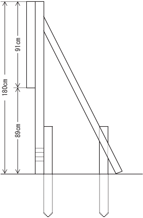
（側面図）
