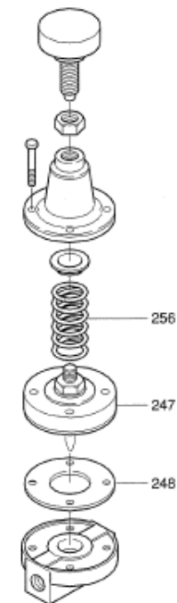
圧力調整弁 246
