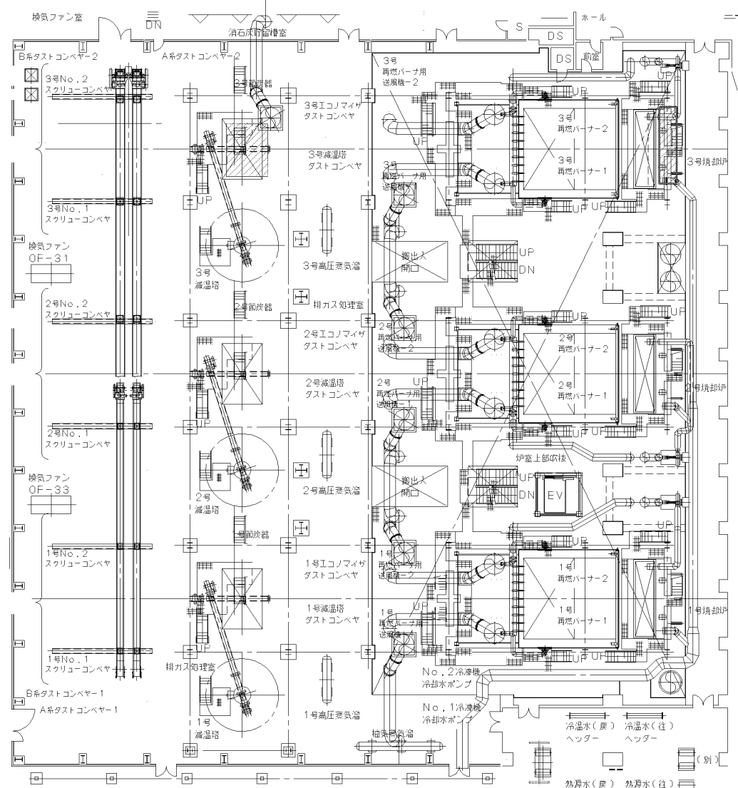
エコノマイザ下M/H 給じん装置 (3階)
