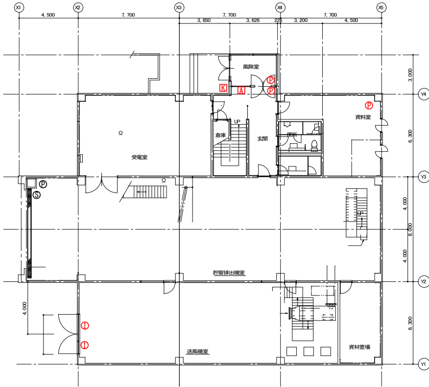
平面詳細図(1階) 1/200
