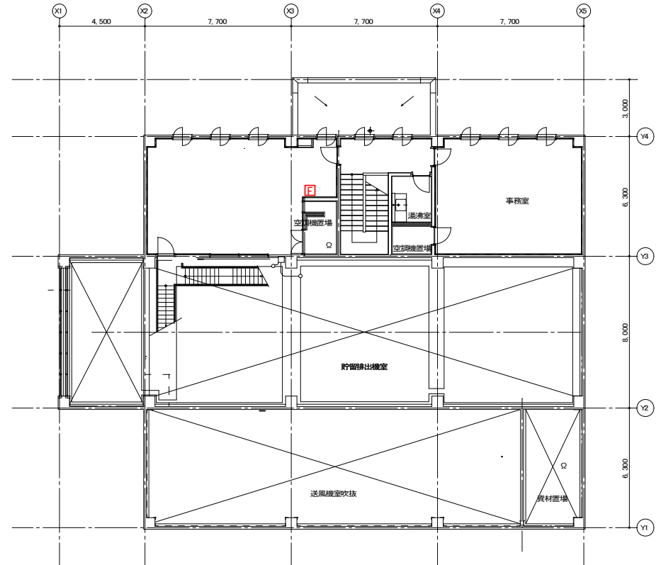
平面詳細図(2階) 1/200
