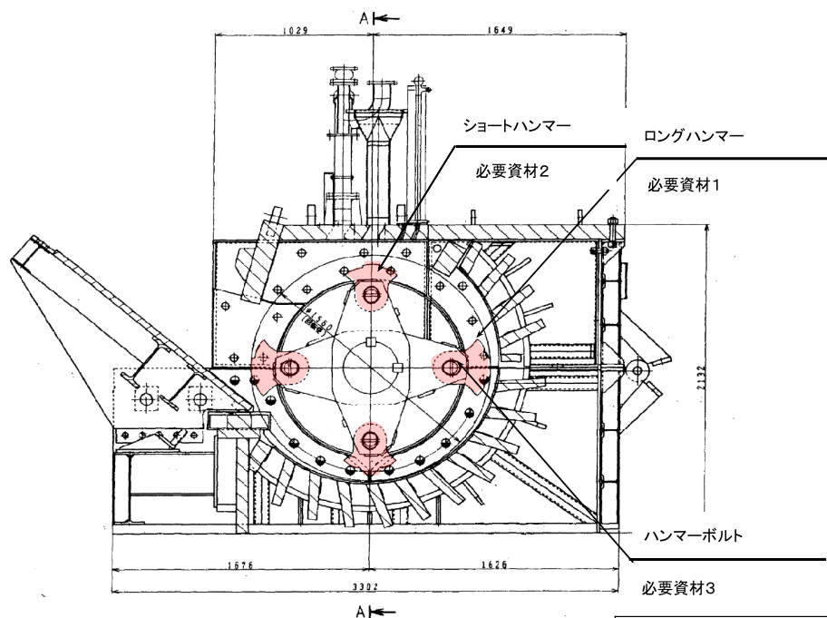
断面 A-A
