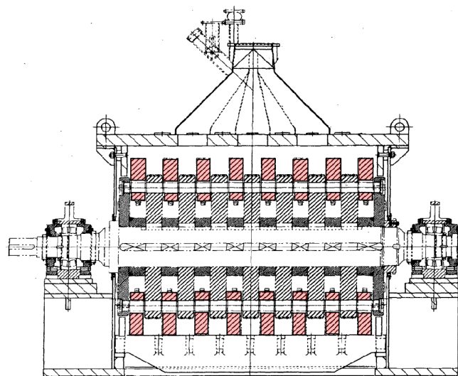
断面 A-A
