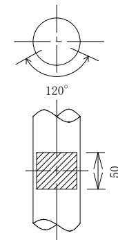
肉厚測定範囲図
