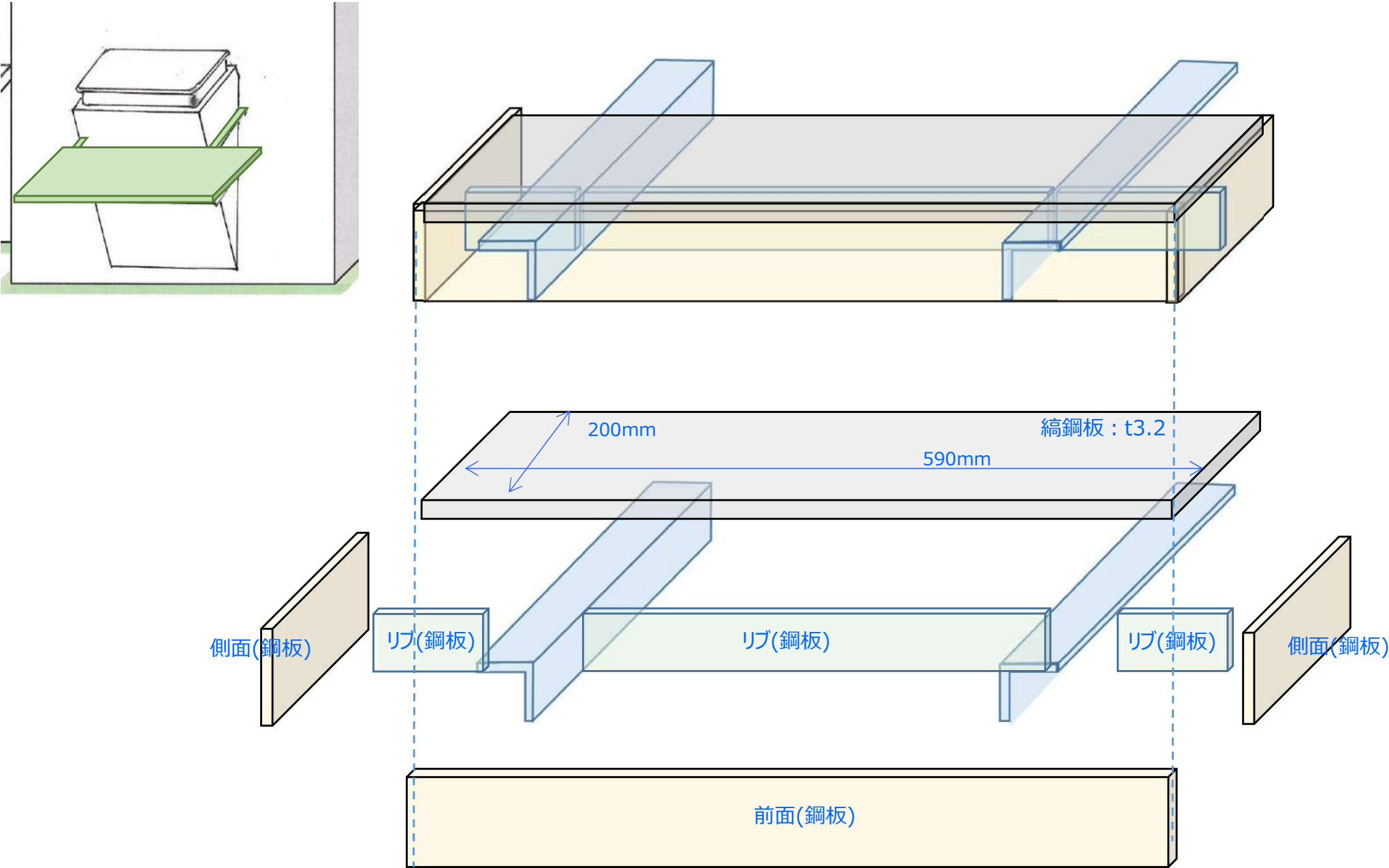
別図③足場形状
