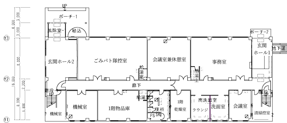
1 階平面図
