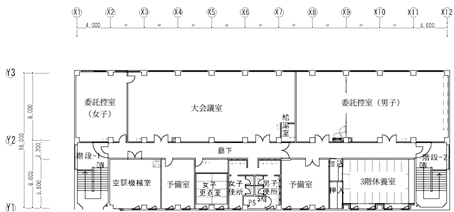
3 階平面図
