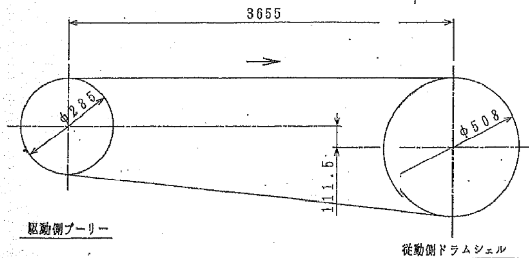
アルミ精選機樹脂ベルト(参考図)
