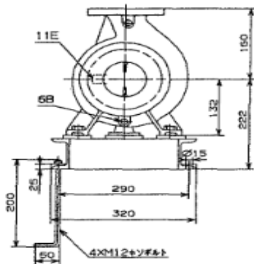
吸込側フランジ
