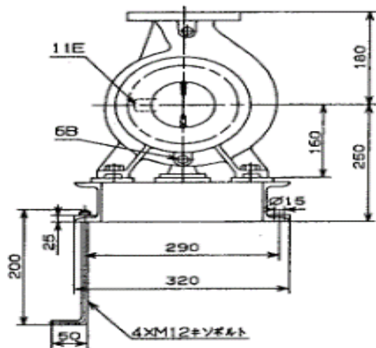
吸込側フランジ
