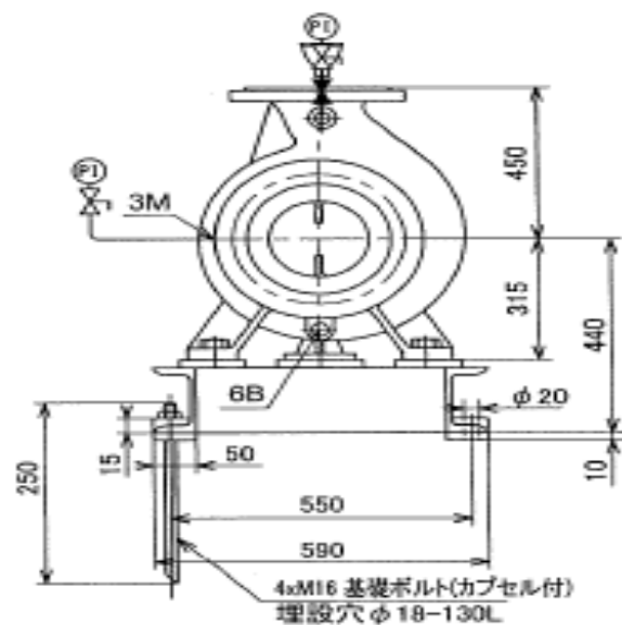
吸込側フランジ JIS 10K RF 200A
