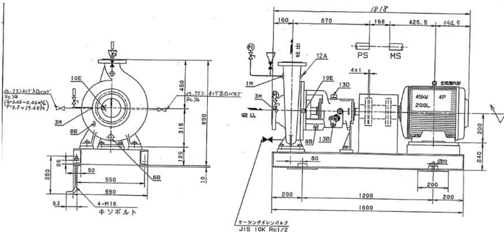
吸込側フランジ JIS 10K RF 200A
