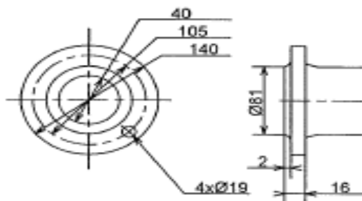
吐出し側フランジ JIS 10K RF 40A
