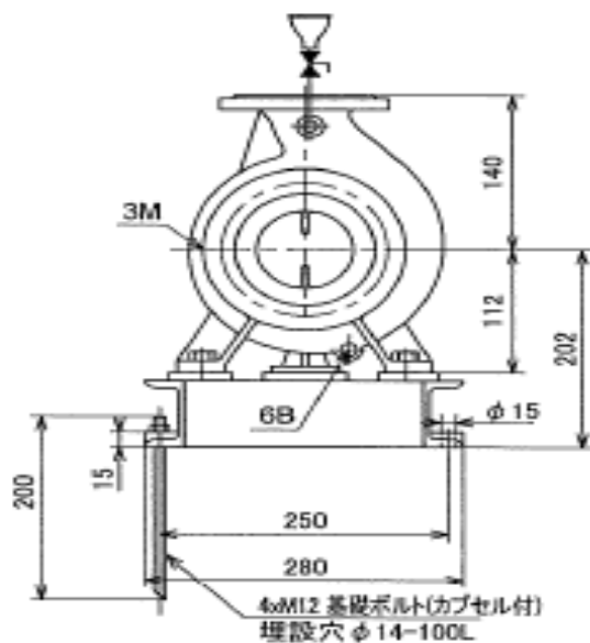
吸込側フランジ JIS 10K RF 65A
