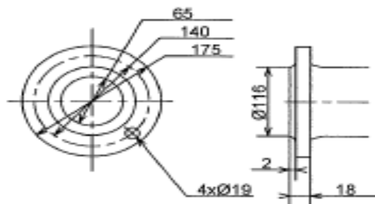
吸込側フランジ JIS 10K RF 65A
