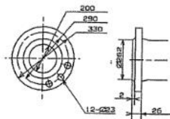
吸込側フランジ JIS 10K RF 200A
