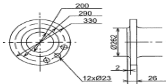
吸込側フランジ JIS 10K RF 200A
