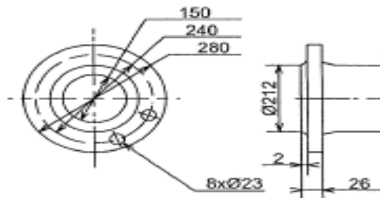
吐出し側フランジ JIS 10K RF 150A
