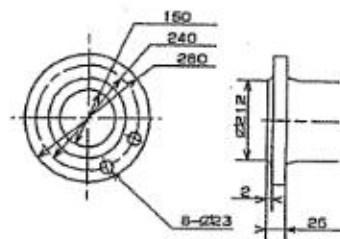
吐出側フランジ JIS 10K RF 150A
