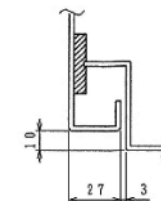
扉詳細図 (1/2)
