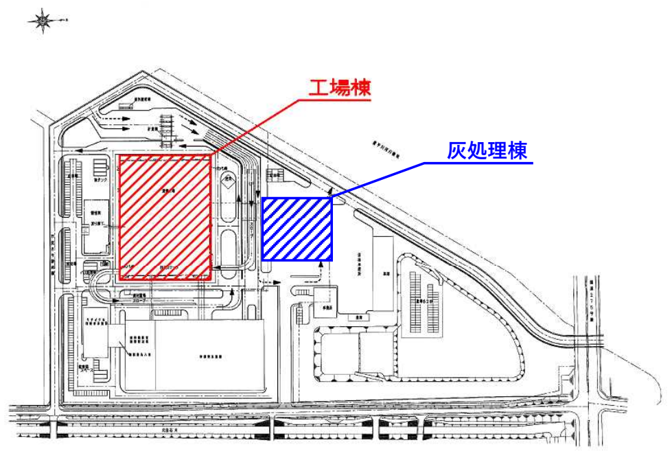
白石清掃工場配置図
