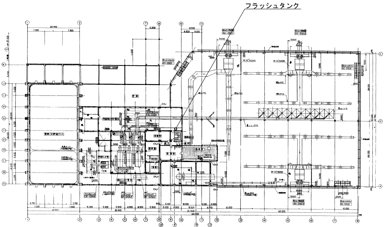
2階平面図
