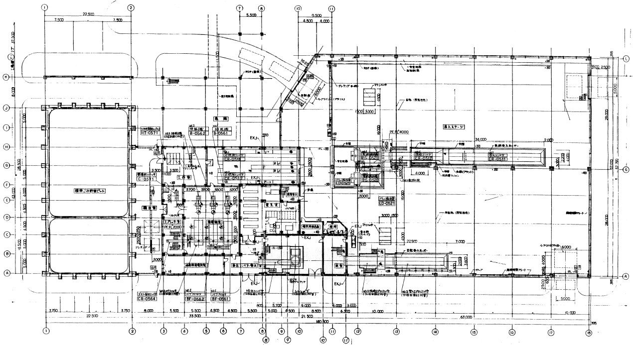
1階平面図
