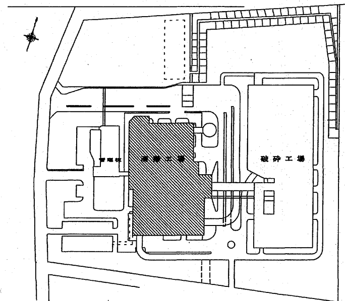
駒岡清掃工場配置図 1 : 3000
