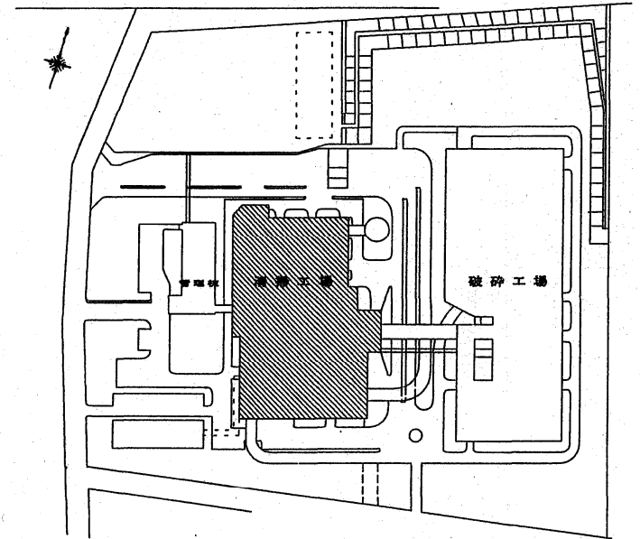
駒岡清掃工場配置図 1 : 3000
